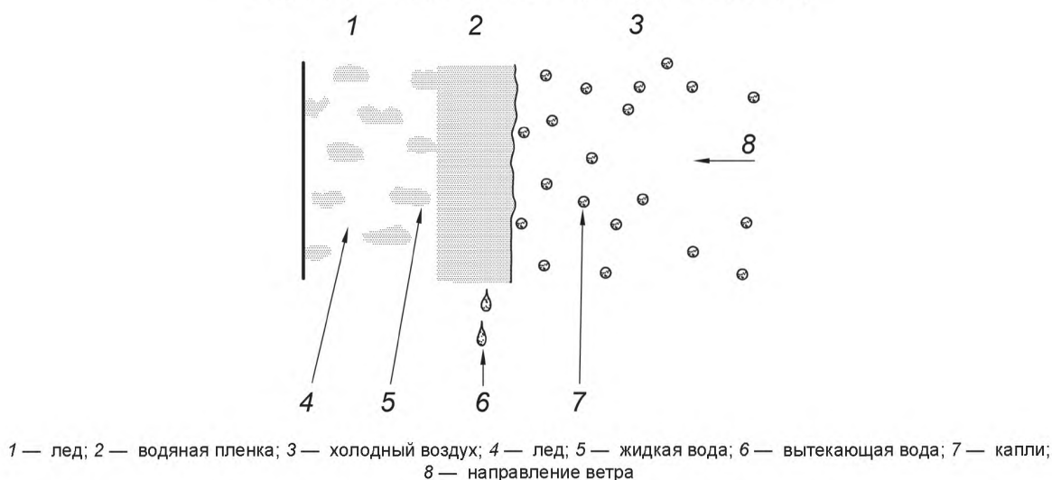
Рисунок С.3 — Образование гололеда («влажный прирост»)
