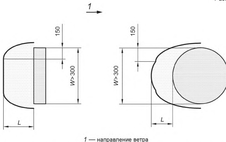
Рисунок 5 — Модель изморозевого обледенения для больших объектов
