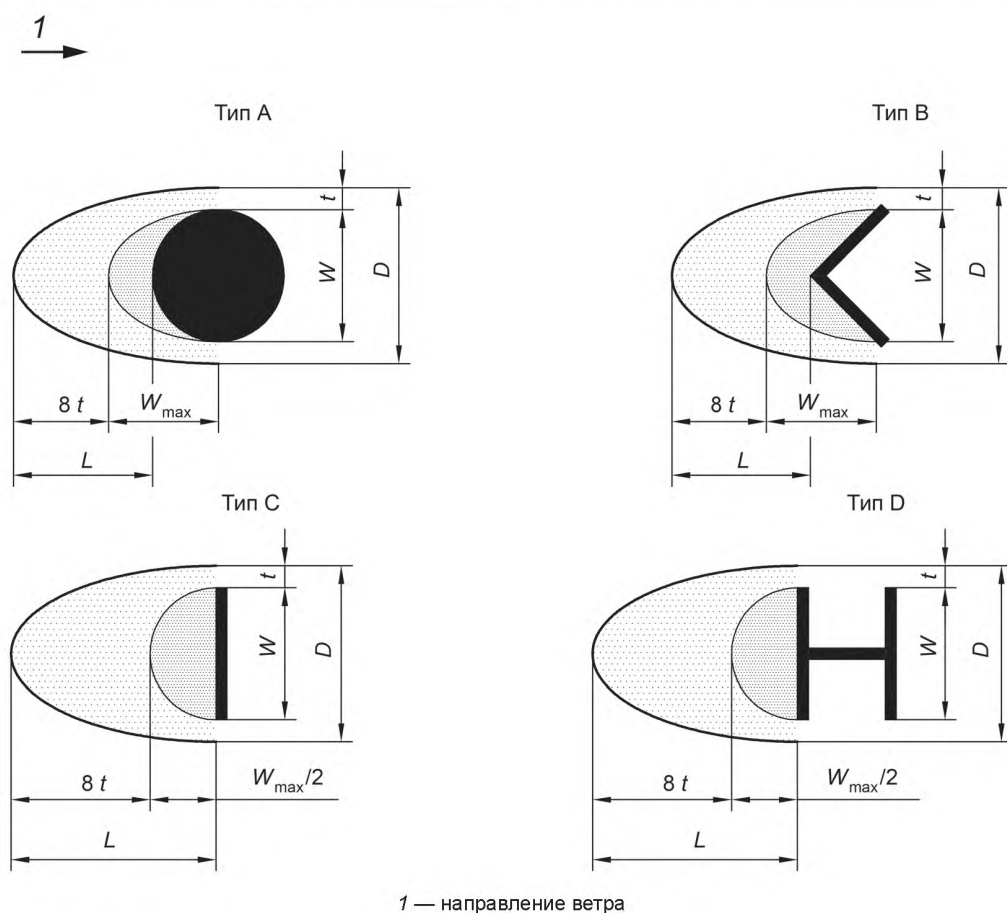
Рисунок 4 — Модель изморозевого обледенения (лист 1)
