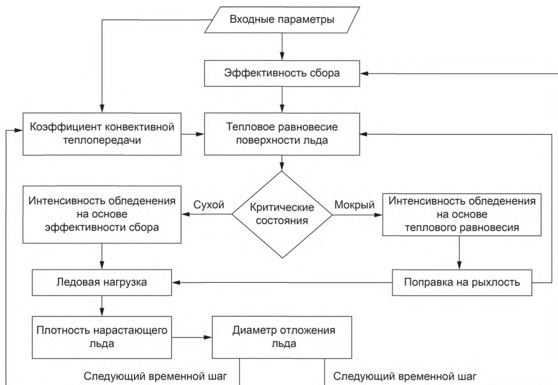
Рисунок С.5 — Упрощенная блок-схема численной модели обледенения
