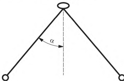
Рисунок К.3 — Графическое представление подъемного узла, показывающее угол отклонения стропа от вертикали
