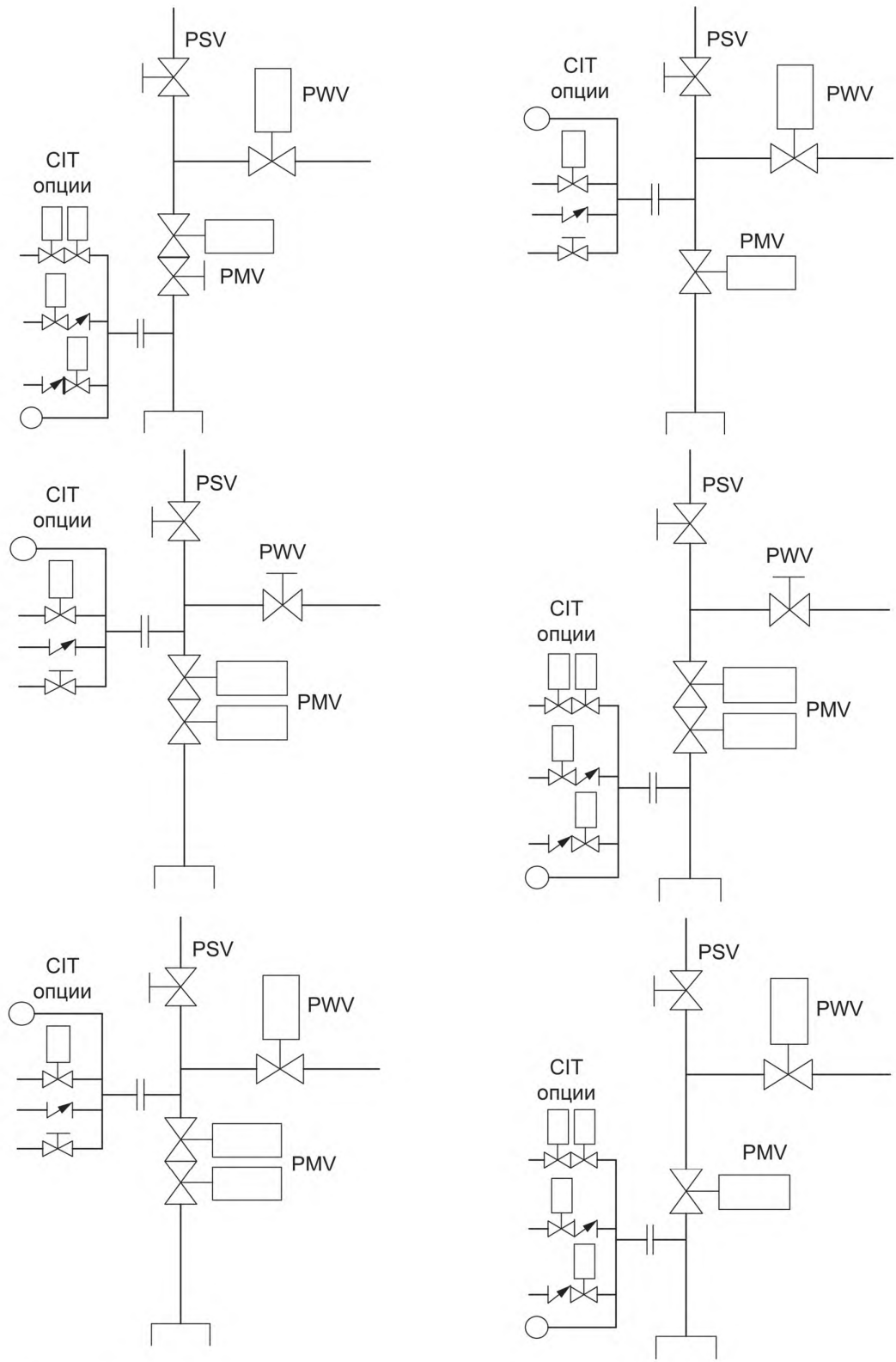
а) Примеры проходов (пенетраций) эксплуатационных каналов
