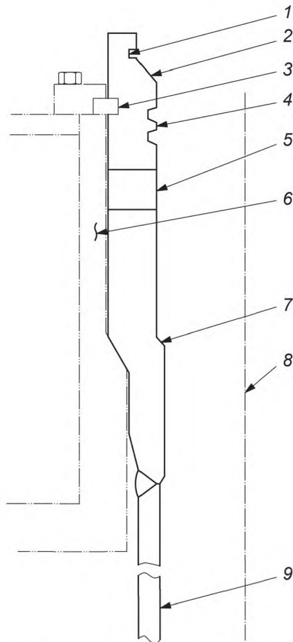
1 — запирающее устьевое оголовка; 2 — посадочный запялик для устьевое оголовка; 3 — крепление постоянной донной направляющей плиты; 4 — подготовка спуско-подъемного инструмента и соединителя колонны-надставки; 5 — цементный порт (опционально); 6 — постоянная донная направляющая плита; 7 — посадочный запялик; 8 — осевая линия; 9 — кондукторная обсадная колонна
