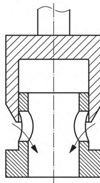
f) Клетка и наружная втулка
