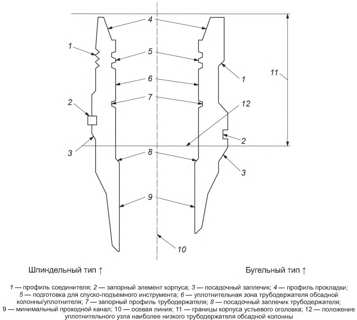
Рисунок 14 — Типовые корпуса устьевых оголовков
