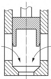
c) Пробка и клетка
