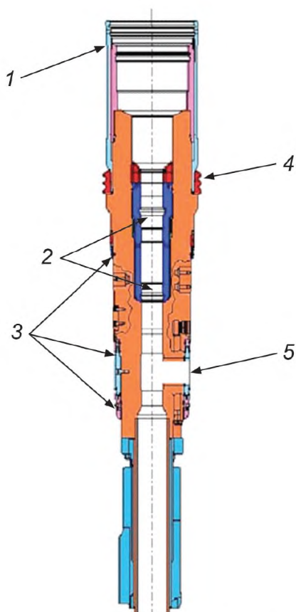
Рисунок D.4 — Трубодержатель НКТ расширенной конфигурации устьевой елки горизонтального типа
