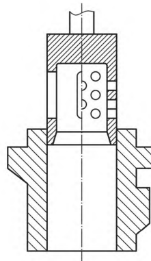
d) Скользящая втулка и клетка
