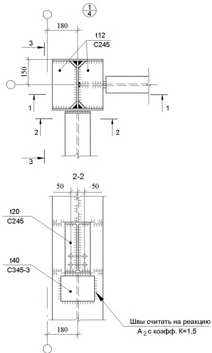
Рисунок К.1 — Пример выполнения чертежа узла металлической конструкции
