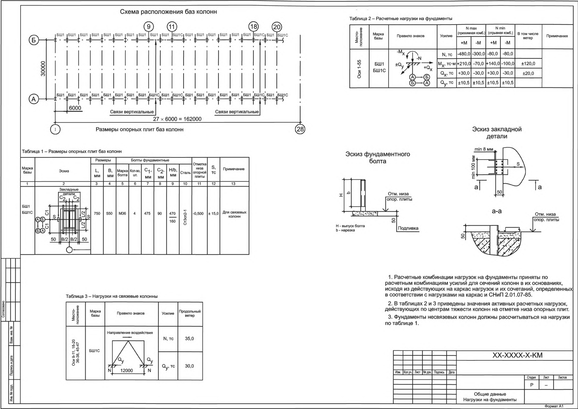
Рисунок В.1 — Пример выполнения нагрузок на фундаменты
