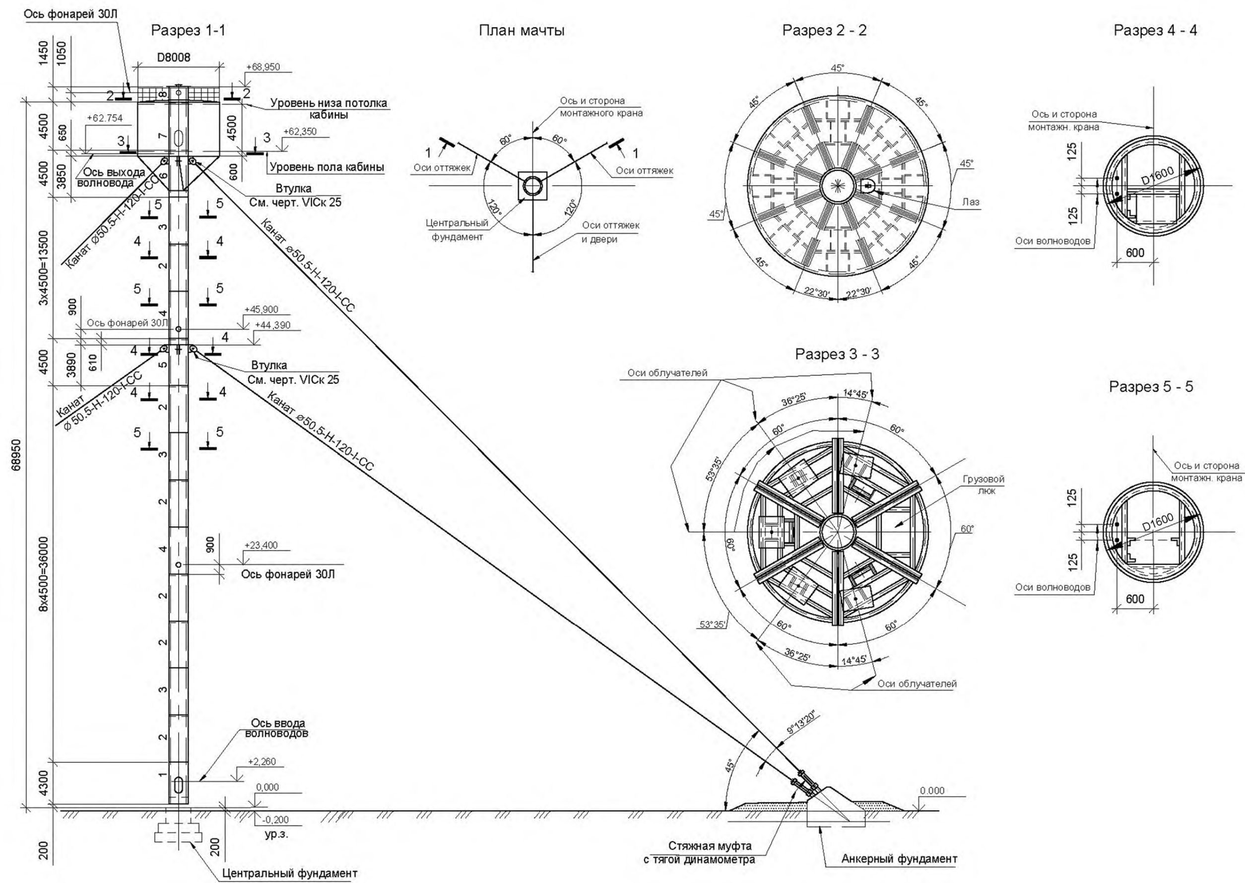
Рисунок Г.2 — Пример выполнения чертежа общего вида мачты
