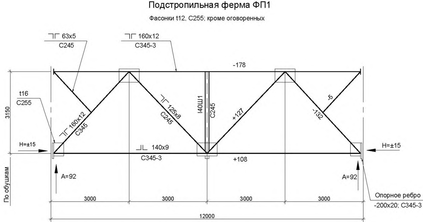
Рисунок И.1 — Пример выполнения чертежа элемента металлической конструкции
