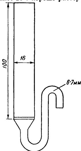
Рис. 11. Хроматографическая колонка
