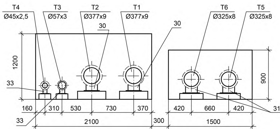
Рисунок Г.1 — Поперечный разрез при подземной прокладке
