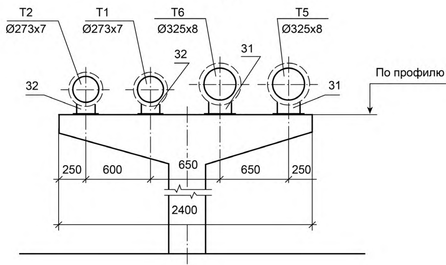
Рисунок Г.2 — Поперечный разрез при надземной прокладке
