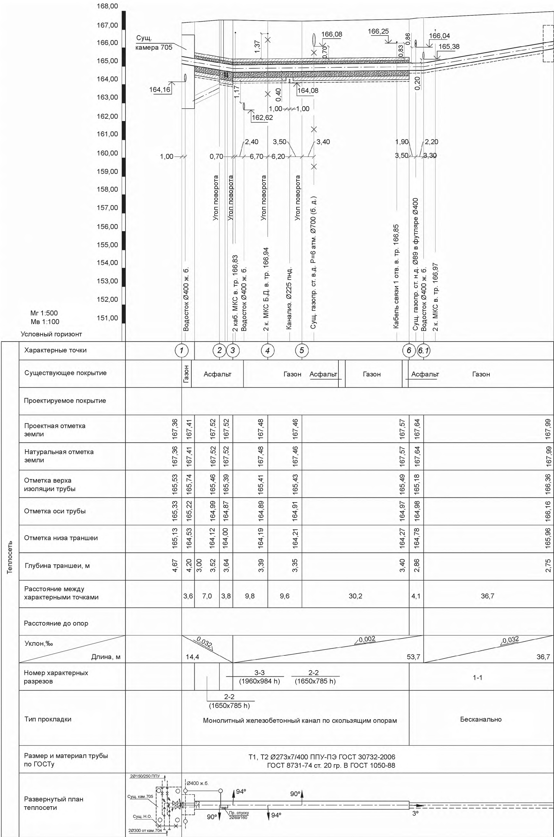
Рисунок Д.2 – Пример оформления продольного профиля бесканальной прокладке
