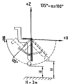
Рис. 1. Наклон пассажирских кресел вперед
