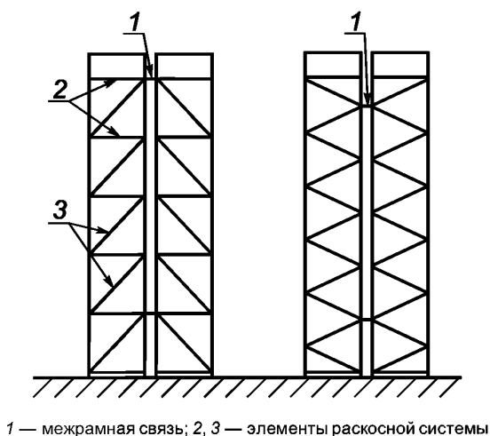
Рисунок 17 — Схема установки межрамных связей
