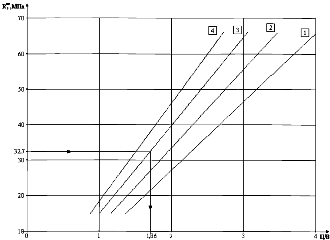
Рисунок 4.1 – Зависимость прочности бетона через 28 суток нормального твердения от Ц/В отношения и класса прочности цемента; 1 – цемент ЦЕМ 22,5; 2 – цемент ЦЕМ 32,5; 3 – цемент ЦЕМ 42,5; 4 – цемент ЦЕМ 52,5
