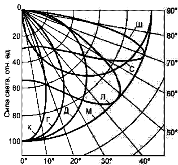
Рисунок 1.6 – Типовые кривые силы света по ГОСТ Р 54350
