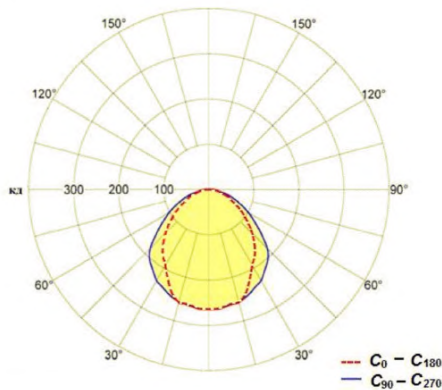
Рисунок Б.1 – Кривая силы света светильника с симметричным светораспределением
