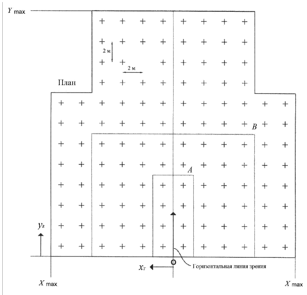
Рисунок 2.3 – Стандартное расположение светильников в плане помещения (Площадь А соответствует размерам 2Н×4Н, площадь В соответствует размерам 8Н×6Н)
