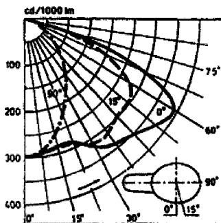
Рисунок 1.7 – Пример представления КСС несимметричного светильника в каталогах
