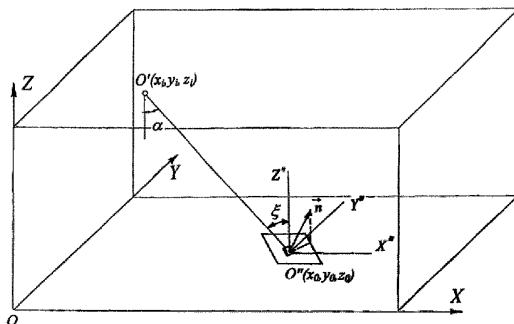
Рисунок 1.9 – Привязка помещения и светильников к осям координат
