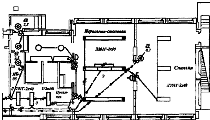
Рисунок 3.9 – Схема размещения светильников в ячейке детского сада-яслей
