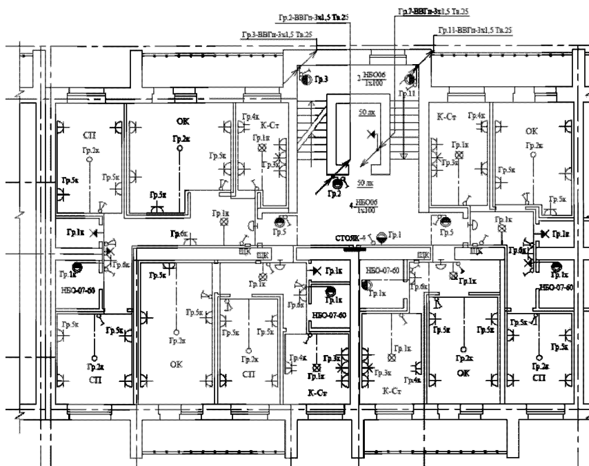
Рисунок 4.1 – Искусственное освещение секции жилого дома
