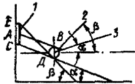
Рисунок 3.4 – Расположение зеркальной вставки:
