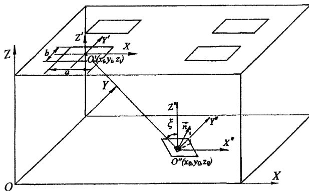
Рисунок 1.14 – К расчету освещенности от прямоугольного излучателя
