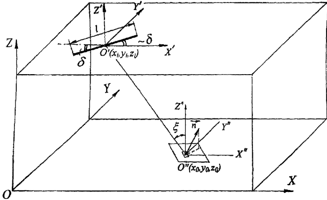
Рисунок 1.13 – К расчету освещенности от линейного излучателя
