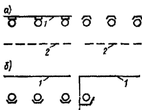
Рисунок 3.1 – Основные светотехнические схемы светящихся потолков:
