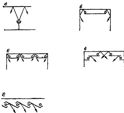
Рисунок 3.2 – Способы устройства отраженного освещения:
