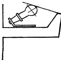
Рисунок 3.6 – Использование зеркальных ламп в световых карнизах
