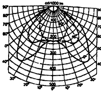
Рисунок 1.8 – Пример представления КСС несимметричного светильника в каталогах
