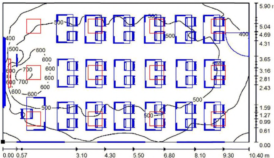
Рисунок 3.10 – Схема размещения светильников в классе
