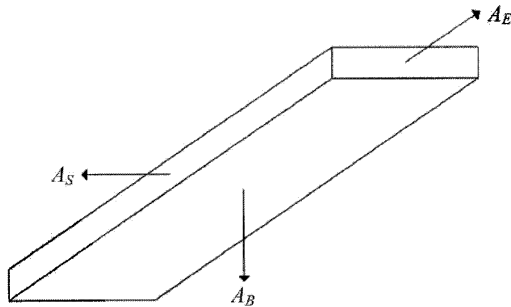
Рисунок 2.2. Расположение светящихся поверхностей светильника, видимых работающим в помещении
