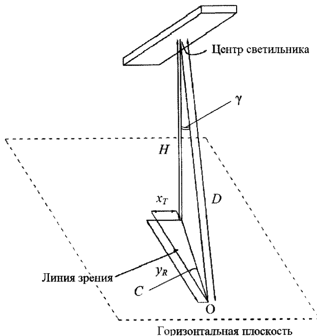
Рисунок 2.1 – Расположение центра светильника относительно работающего
