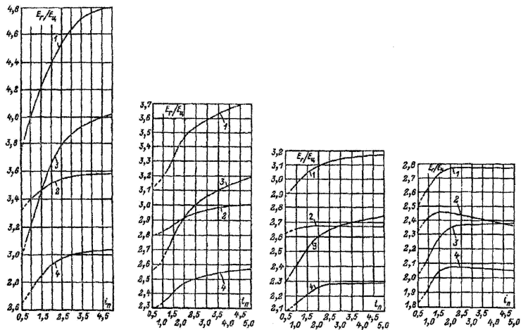
Рисунок 2.5 – Графики для расчета цилиндрической освещенности
