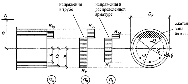
Рисунок 7.3 – Схема усилий и эпюра напряжений в сечении, нормальном к продольной оси внецентренно сжатого трубчатобетонного элемента, при расчете его по прочности
