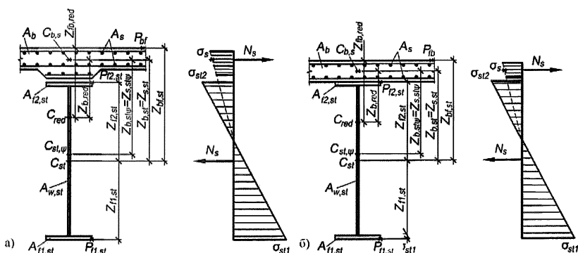
а) плита с вутами; б) плита без вут
