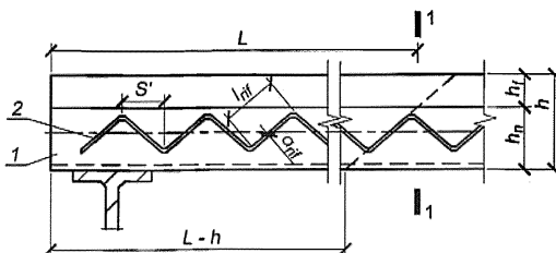
Рисунок 6.9 – Схема усилий при расчете по прочности анкеровки
