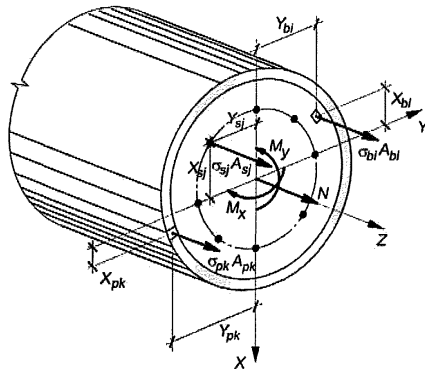
Рисунок 7.4 - Расчетная схема нормального сечения трубобетонного элемента
