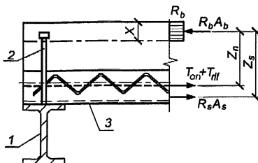
Рисунок 6.9 – Схема усилий при расчете по прочности анкеровки
