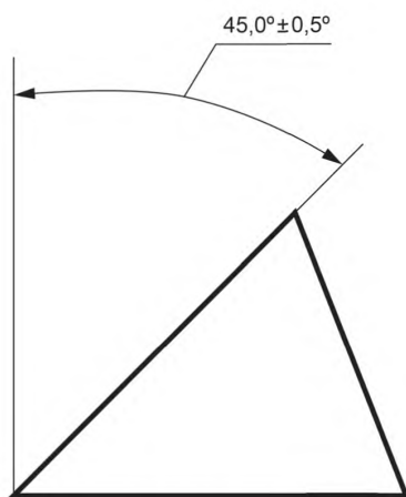
Рисунок 4 — Схема оправки
