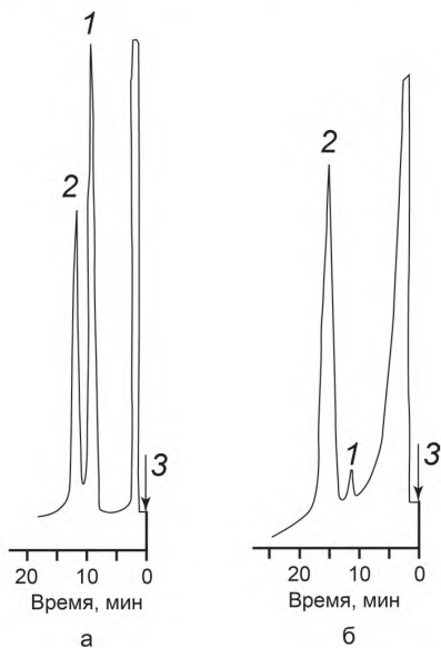
1 — фенол; 2 — м-крезол; 3 — ввод пробы
