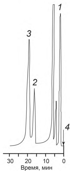
1 — ацетон; 2 — фенол; 3 — м-крезол; 4 — ввод пробы
