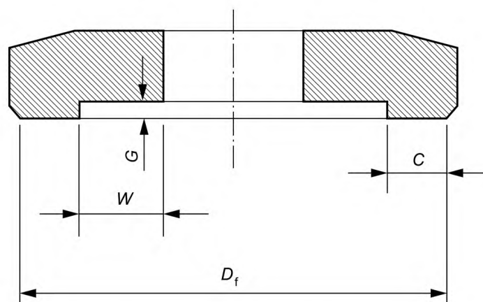
b) конструкция фланца, пример b)
