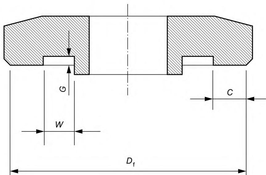
a) конструкция фланца, пример а)
