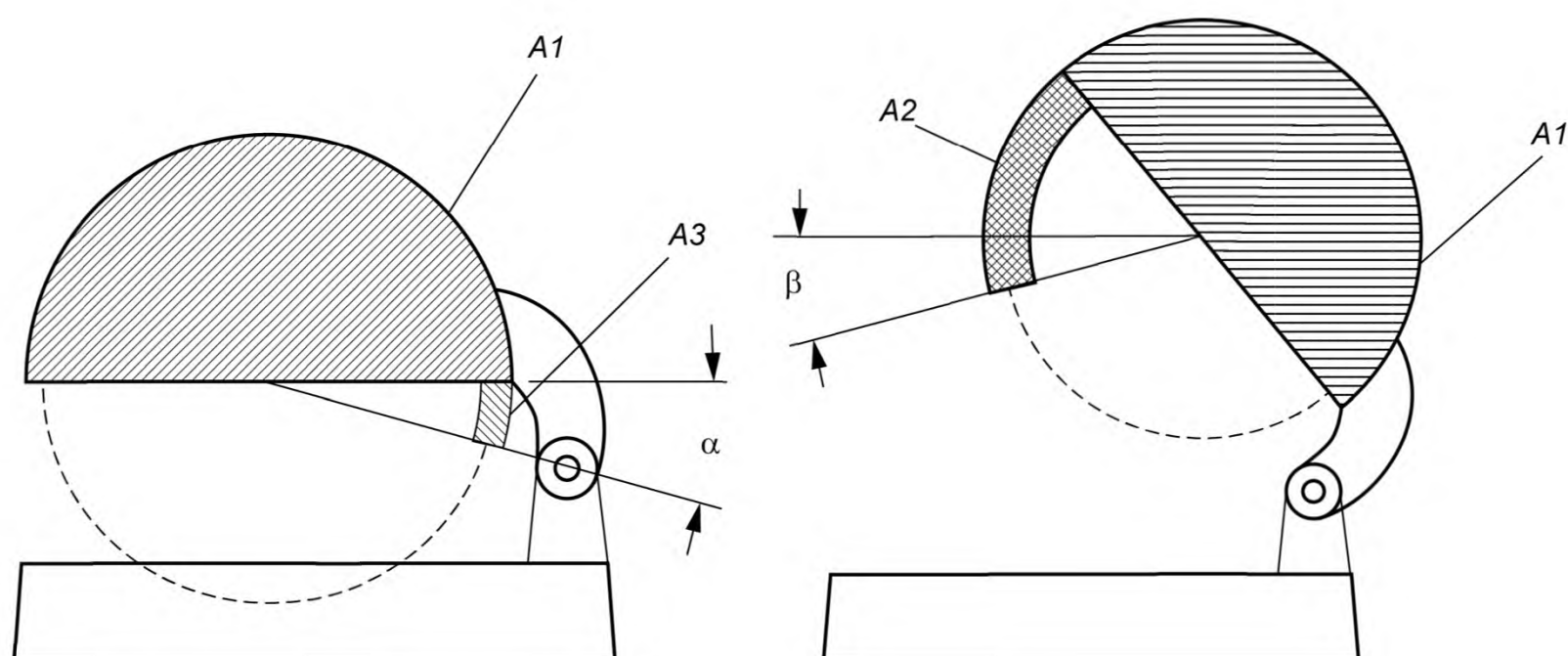
а) Режущая головка в самом нижнем положении
