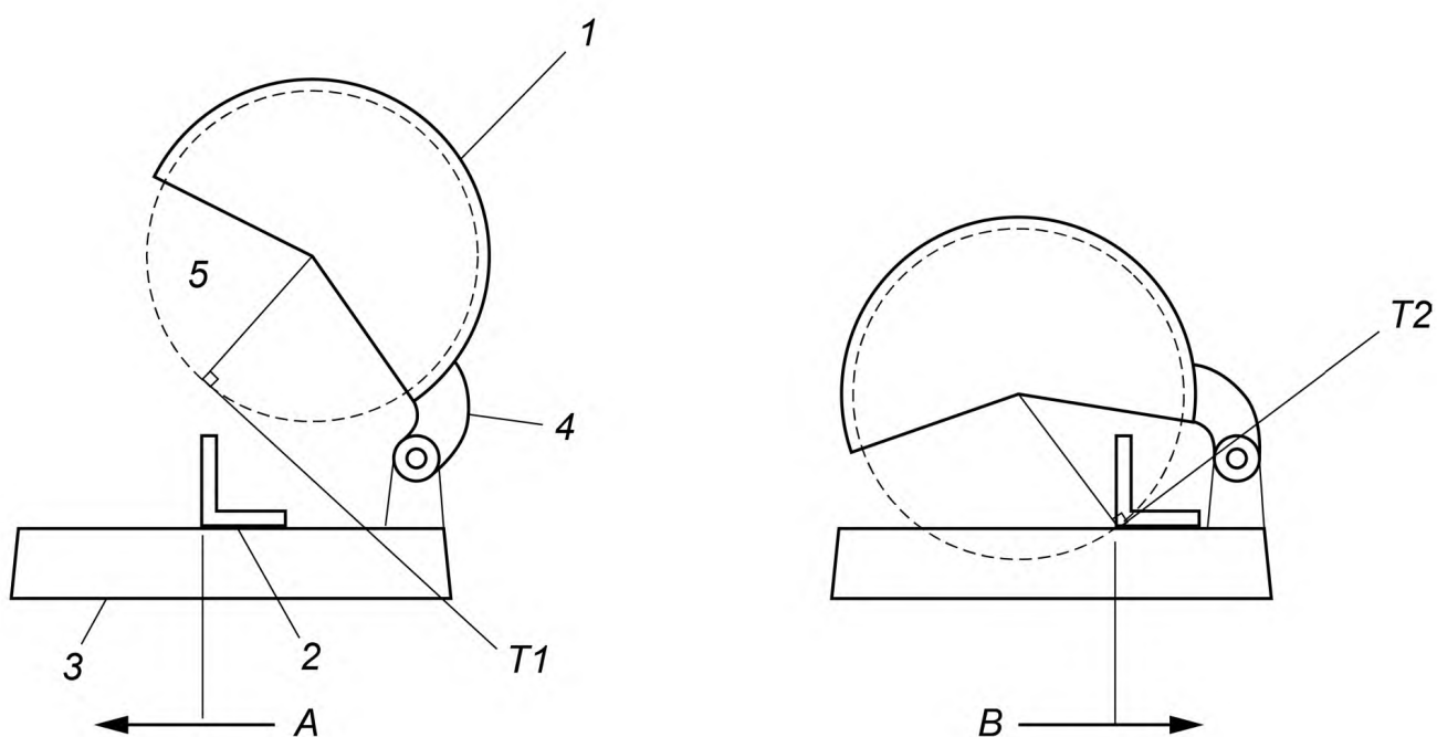
Рисунок 104 — Испытательный щуп
