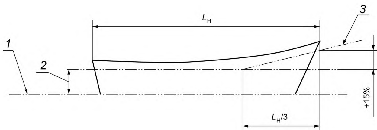
Рисунок 4 — Требуемая минимальная высота заливания — проектная категория D.
