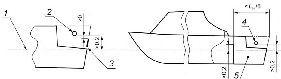
1 — ватерлиния; 2 — отверстие со степенью водонепроницаемости 3 или 4; 3 — шпигат; 4 — отверстие со степенью водонепроницаемости 4; 5 — небыстроосушаемые помещения
