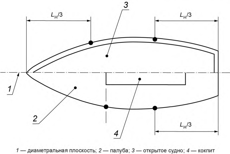
Рисунок Ф.1 — Расположение испытательных грузов
