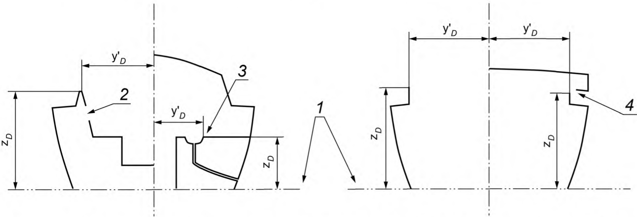
1 — ватерлиния; 2 — отверстия, считающиеся открытыми, защищенные комингом; 3 — пример внутреннего отверстия, считающегося открытым; 4 — пример воздухозаборника двигателя
