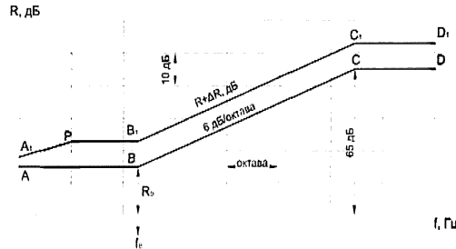
Рисунок 6 - Построение частотной характеристики изоляции воздушного шума стеной с гибкой плитой на относе
