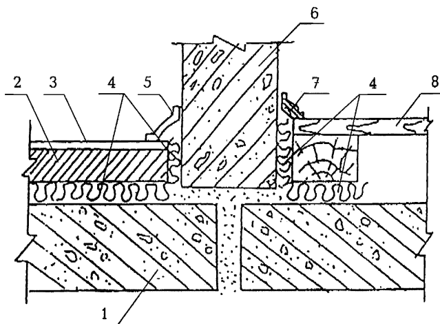
1 – несущая часть междуэтажного перекрытия; 2 – бетонное основание пола 5 – гибкий пластмассовый плинтус; 6 – стена; 7 – деревянная галтель; 8 – дощатый пол на лагах
