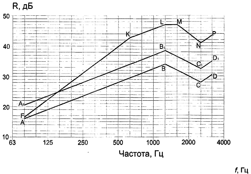
Рисунок А.2 - Расчетная частотная характеристика
