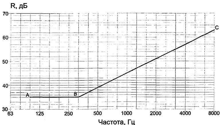
Рисунок А.1 - Расчетная частотная характеристика
