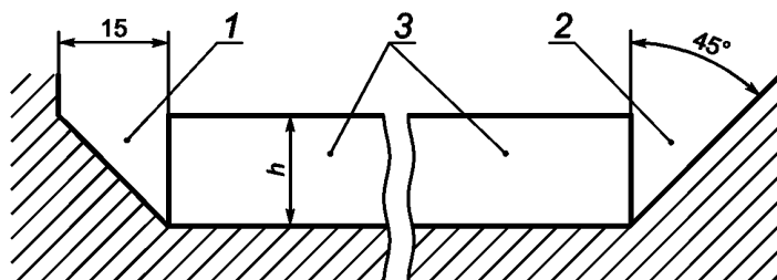
1 — «не препятствующая» зона для лыжных тормозов с тормозным приспособлением (хвостовые лопатки) в направлении носка лыжи; 2 — «не препятствующая» зона для лыжных тормозов с тормозным приспособлением (хвостовые лопатки) в направлении пятки лыжи (или в направлении чехла носка лыжи или иных конструкций); 3 — лыжа; h — 20 мм для лыж для взрослых; h — 18 мм для лыж для детей
