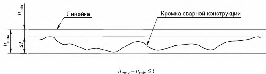
Рисунок 6 — Испытание на прямолинейность
