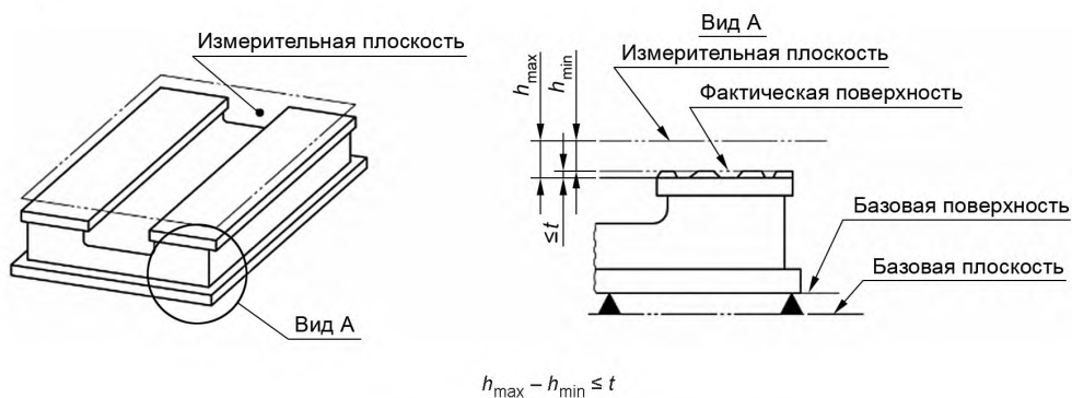
Рисунок 8 — Испытание на параллельность
