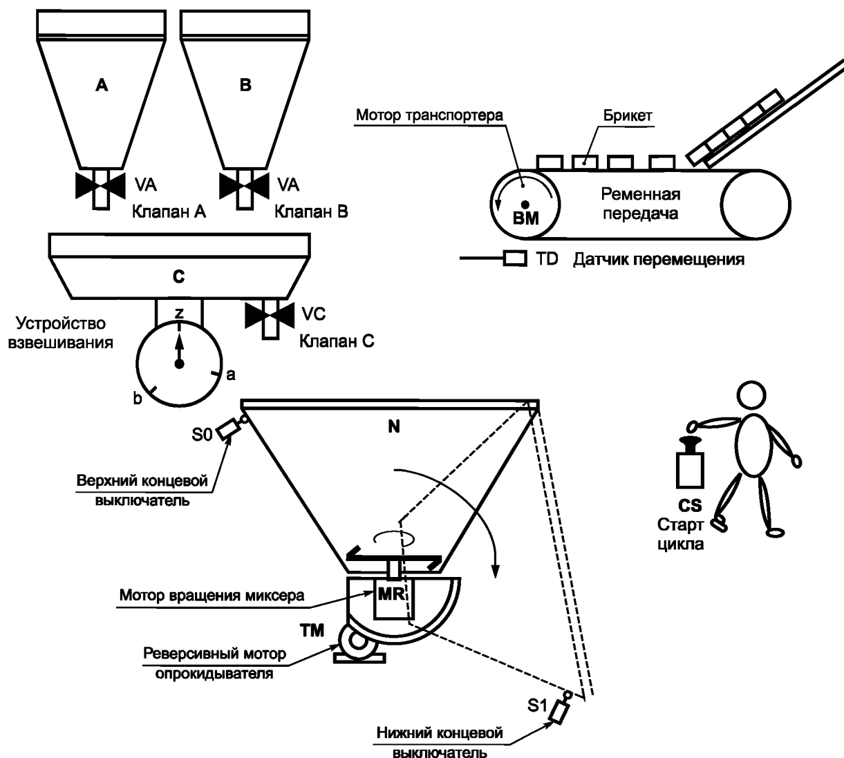
Рисунок В.1 — Структурная схема системы взвешивания-смешивания
