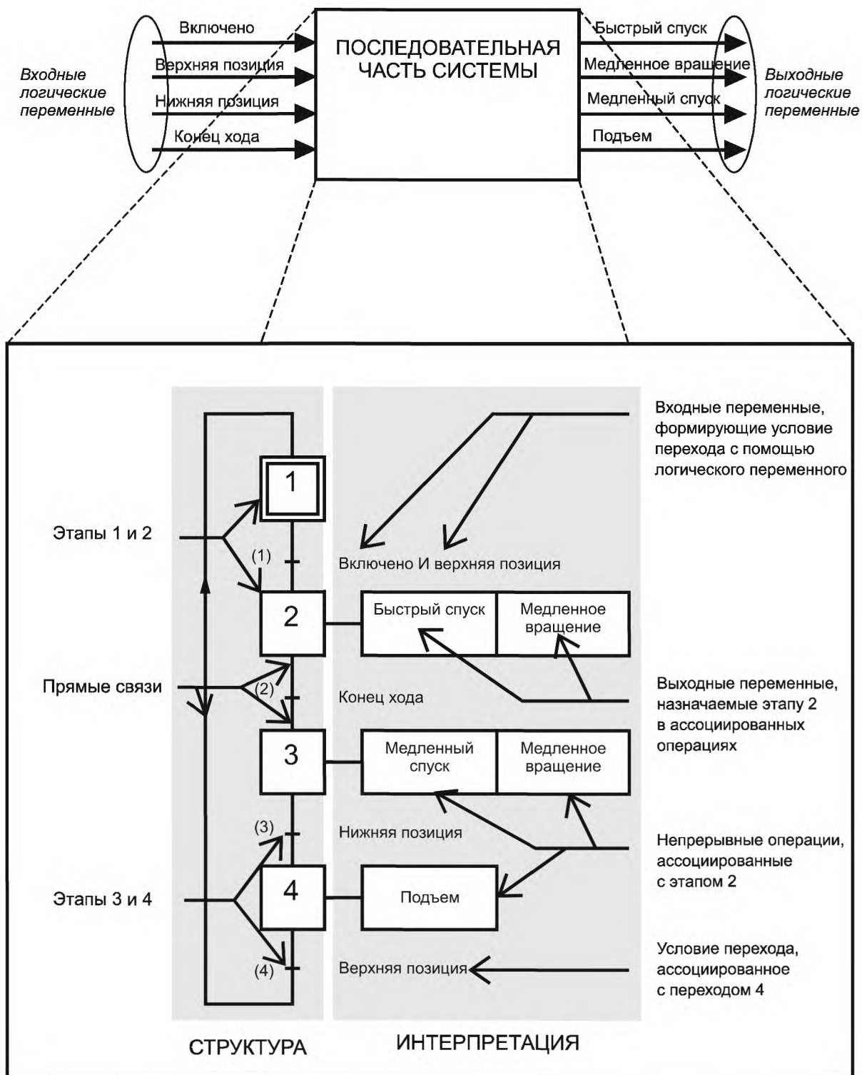
Рисунок 2 — Элементы структуры и интерпретации, используемые в диаграмме grafset для описания поведения последовательной части системы, определяемой ее входными и выходными переменными
