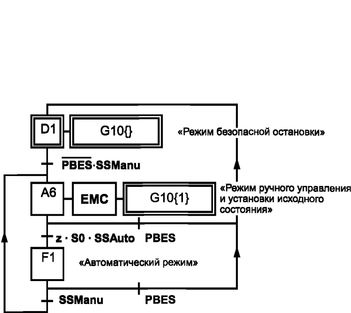
G1: Парциальная диаграмма grafcet режима эксплуатации (верхний иерархический уровень)
