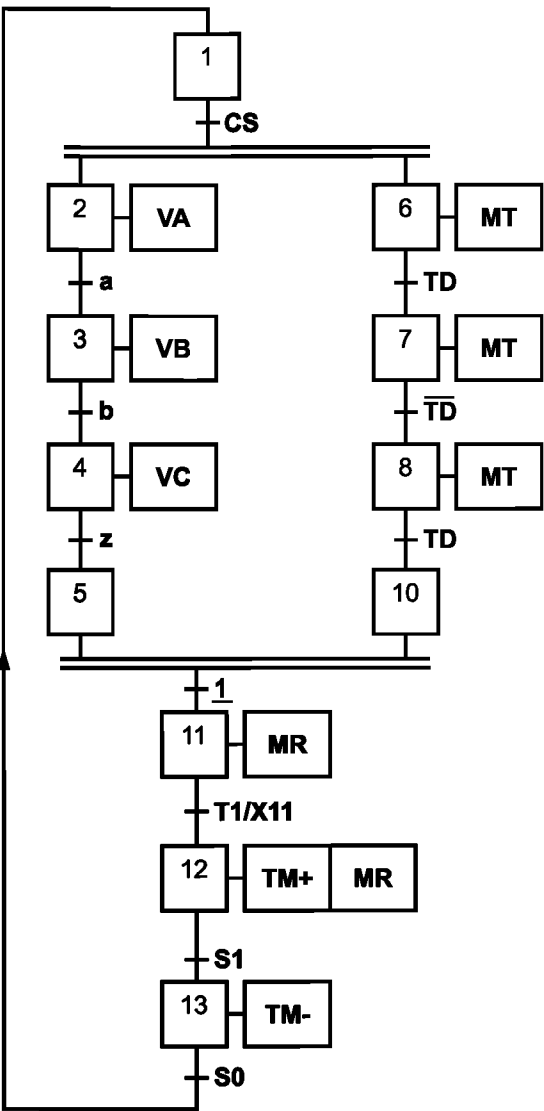
G10: Парциальная диаграмма grafcet автоматического цикла (нижний иерархический уровень)
