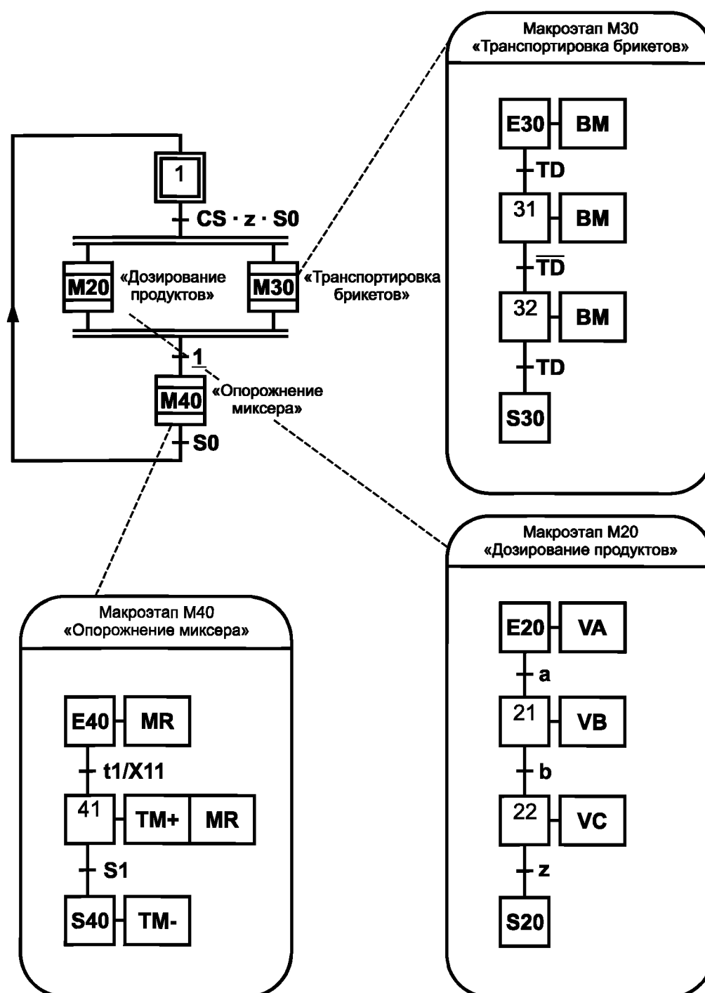
Рисунок В.4 — Диаграмма grafset устройства взвешивания-смешивания с использованием глобального описания на основе макроэтапов и детального описания с помощью расширений макроэтапа
