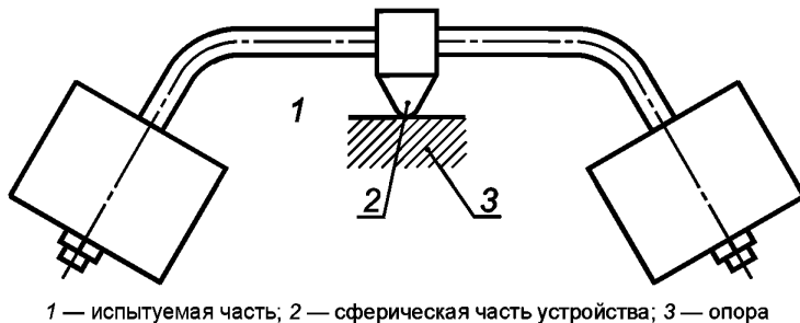
Рисунок 14 — Устройство для испытания давлением шарика
