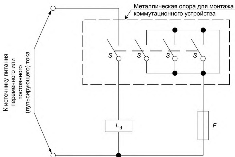
Рисунок 2b — Контактные элементы противоположной полярности, электрически разделенные
