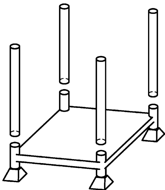
Рисунок А.9 — Разборный стоечный поддон
