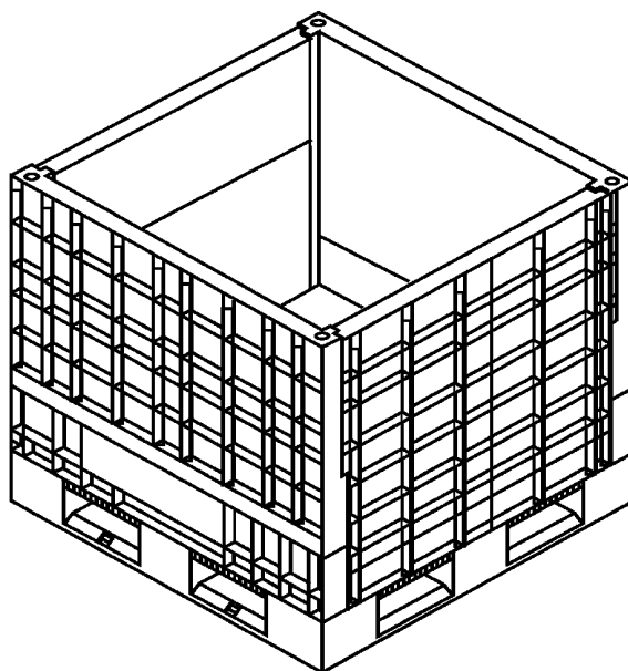
Рисунок А.3 — Ящикный поддон с решетчатыми стенками
