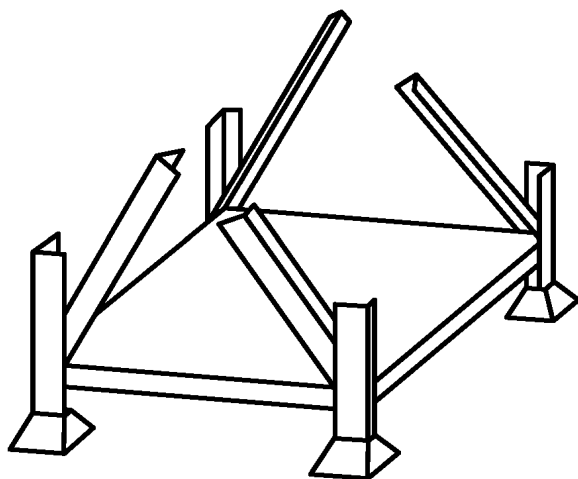
Рисунок А.10 — Складной стоечный поддон
