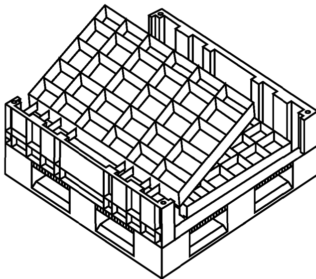
Рисунок А.6 — Складной ящичный поддон с решетчатыми стенками
