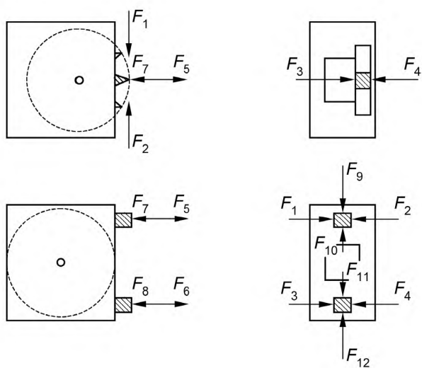
Рисунок 3e — Диск
