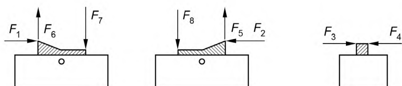
Рисунок 3d — Балансир
