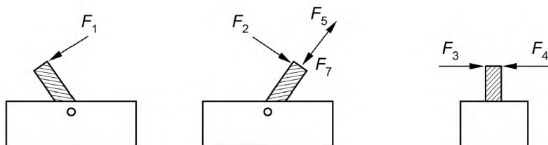
Рисунок 3b — Рычаг
