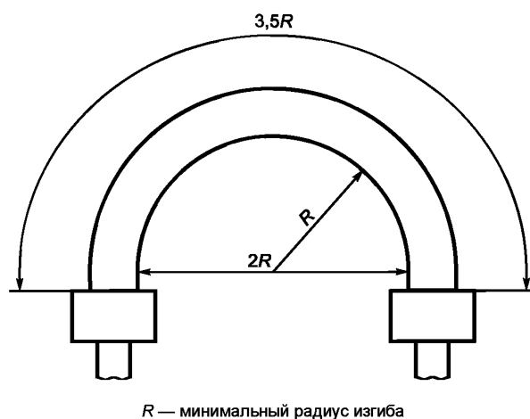
Рисунок 3 — Схема изгиба рукавов при динамических испытаниях
