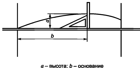
Рисунок 1 — Определение диагонального перекоса
