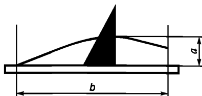
Рисунок 4 — Пример 2 общего диагонального перекоса
