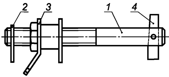
1 — стержень с резьбой; 2 — стопорное устройство; 3 — подвижное устройство с отверстием для закрепления карабином пояса; 4 — падающее на 90° запорное устройство
