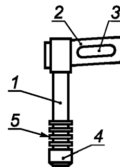
1 — основной стержень из прутка; 2 — флажок для закрепления карабином строительного предохранительного пояса; 3 — отверстие флажка для закрепления карабином строительного предохранительного пояса; 4 — конец приспособления, вставляемый в отверстие ребра жесткости опалубки; 5 — кольцевые выступы
