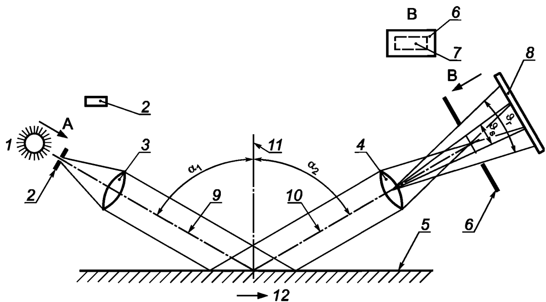
1 — источник света (источник); 2 — апертура источника света; 3 — линза источника света; 4 — линза приемника излучения; 5 — испытуемая поверхность; 6 — полевая диафрагма приемника излучения; 7 — изображение апертуры источника на полевой диафрагме приемника излучения; 8 — приемник излучения; 9 — оптическая ось падающего пучка света; 10 — оптическая ось отраженного пучка света; 11 — нормаль к поверхности испытуемого образца; 12 — направление измерения; \alpha_1 — угол между 9 и 11; \alpha_2 — угол между 10 и 11; \nu_r — угол апертуры приемника излучения; \nu_s — угол апертуры приемника излучения
