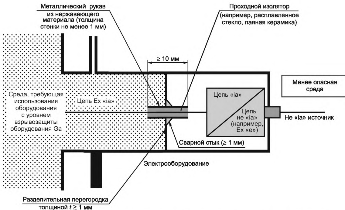
Рисунок 1 — Пример газонепроницаемой разделительной перегородки с проходным изолятором
