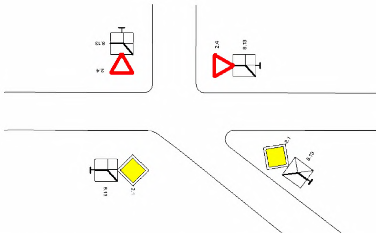
Рисунок Г.1 – Размещение знаков приоритета на главной дороге перед перекрестком, на котором главная дорога изменяет направление
