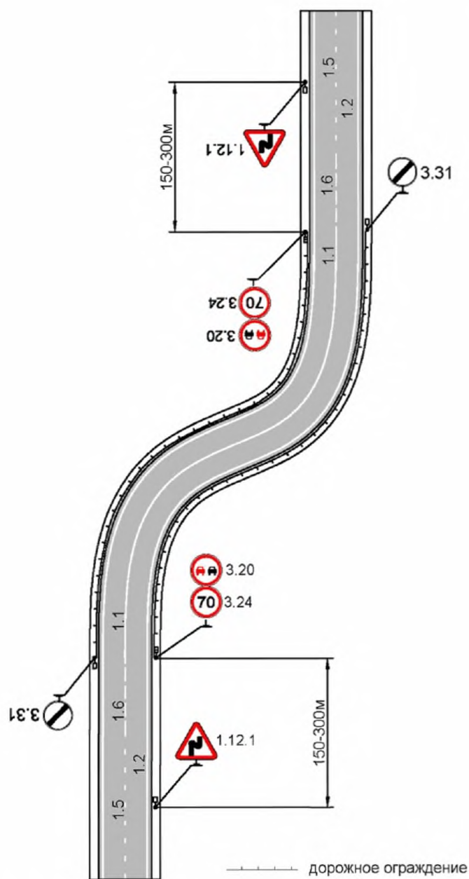
Рисунок Г.23 – Схема организации дорожного движения в зоне двух кривых в плане, следующих друг за другом
