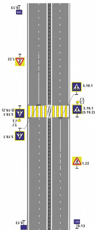
Рисунок Г.11 – Пример применения элементов обустройства при обустройстве нерегулируемого пешеходного перехода вне населенного пункта на дороге с ограждением
