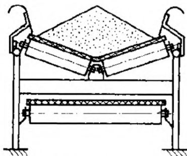
Рисунок 29 – Обычный ленточный конвейер
