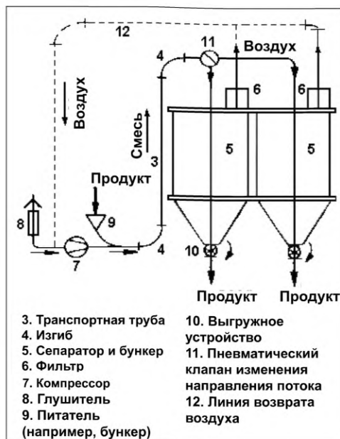
Рисунок 39 – Принцип работы пневматических конвейеров высокого давления
