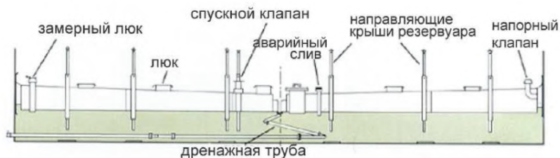
Рисунок 3 – Пример типичной двойной плавающей понтонной крыши
