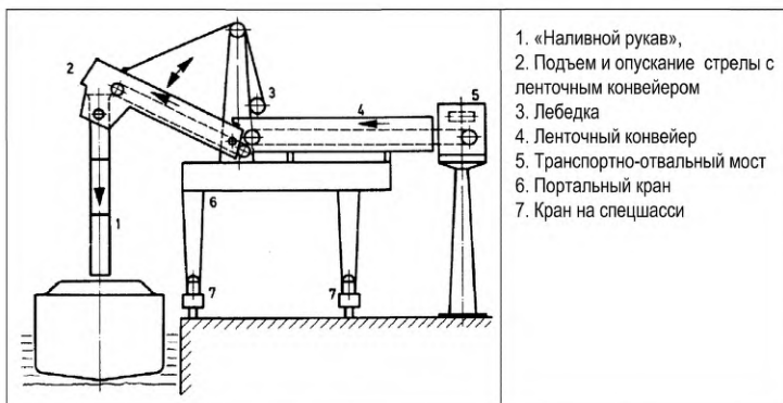
Рисунок 24 – Погрузчик с наливной трубой
