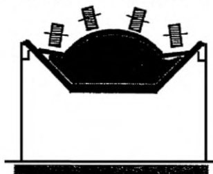
Рисунок 33 – Пример двухленточного конвейера
