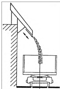
Рисунок 27 – Загрузка вагона с помощью желоба
