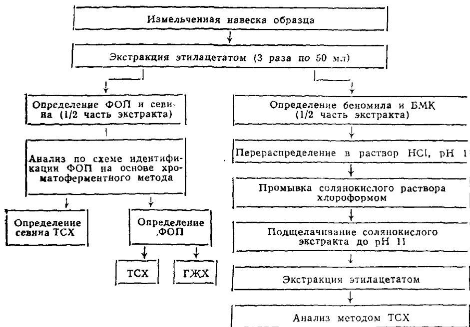
Рис. 15. Схема анализа фосфорорганических пестицидов, севина, беномила и БМК при совместном присутствии.
