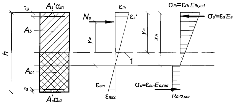
Рисунок 12 – Приведенное поперечное сечение и схема напряженно-деформированного состояния изгибаемого предварительно напряженного элемента с трещинами при его расчете по деформациям
