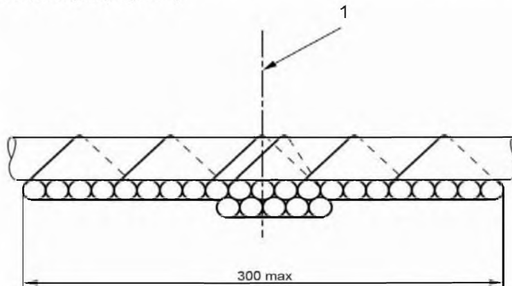
Рисунок 1 – Отрезки кабеля, закрепленные без зазора на передней стороне стандартной лестницы (совокупности отрезков кабеля находятся в непосредственном контакте)
