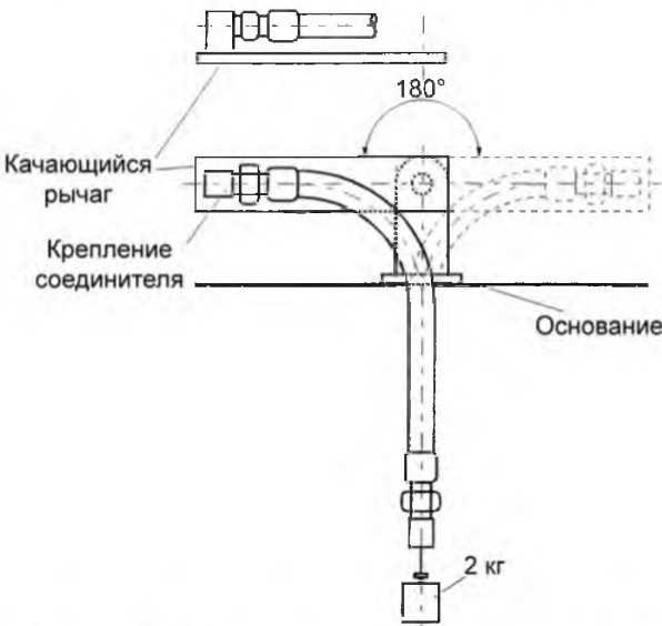
Рисунок 7 – Установка для испытания на гибкость
