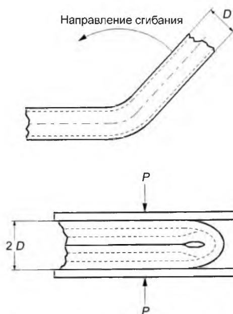
Рисунок 3 – Испытание на перегиб
