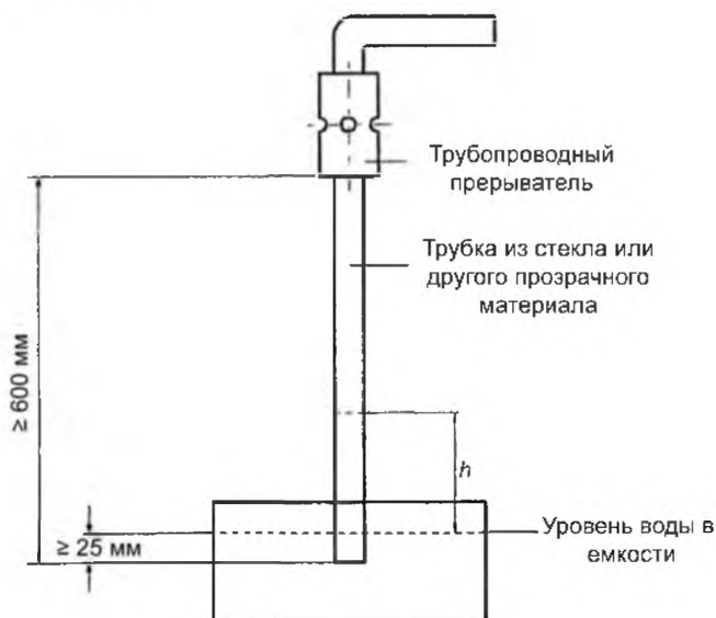
Рисунок 1 – Измерение расстояния h для трубопроводных прерывателей
