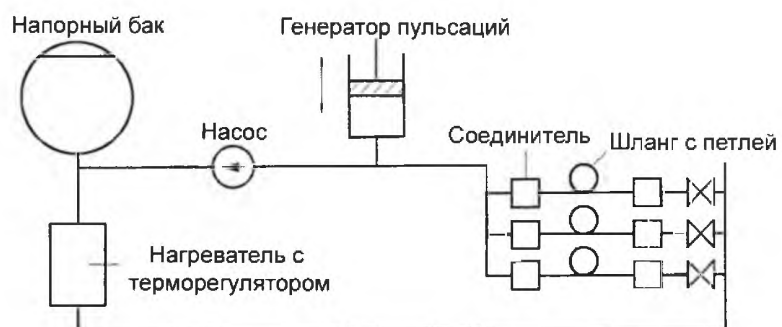
Рисунок 4 – Установка для испытания соединительных шлангов изменяющимся давлением
