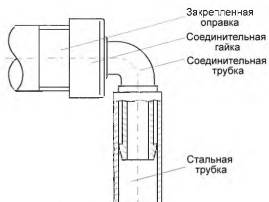
Рисунок 9 – Приложение изгибающего момента к соединительной трубке
