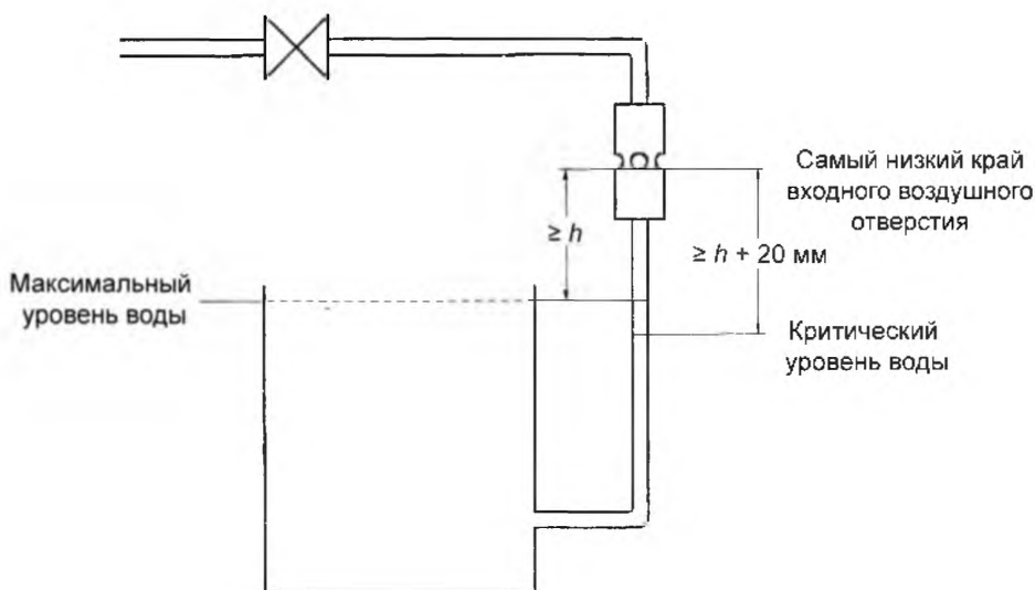
Рисунок 2 – Измерение максимального и критического уровней воды для трубопроводных прерывателей
