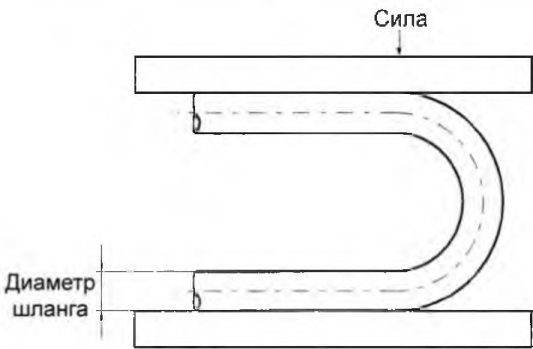
Рисунок 7 – Установка для испытания на гибкость
