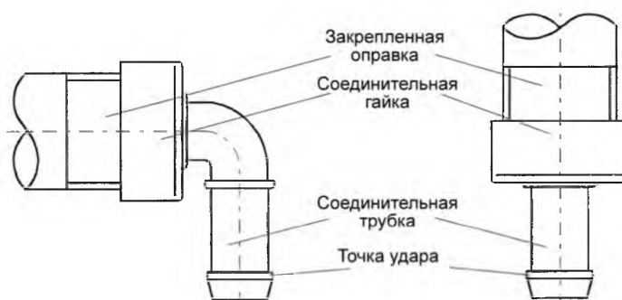
Рисунок 10 – Испытание соединительных трубок ударом
