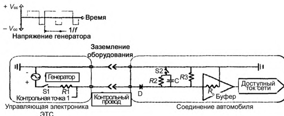
Рисунок В.1 – Типовая цепь управления
