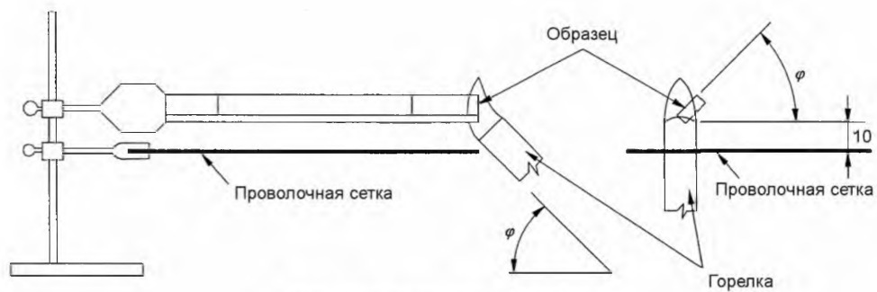
Испытание горизонтального горения
