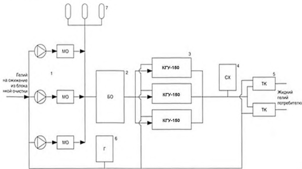
1 – компрессорное отделение с индивидуальной маслоочисткой; 2 – блок осушки; 3 – технологическое отделение (3 уст. КГУ-150); 4 – стационарное хранилище жидкого гелия (120 нм 3 ); 5 – заправка жидкого гелия в транспортные контейнеры; 6 – газгольдеры; 7 – ресиверы
