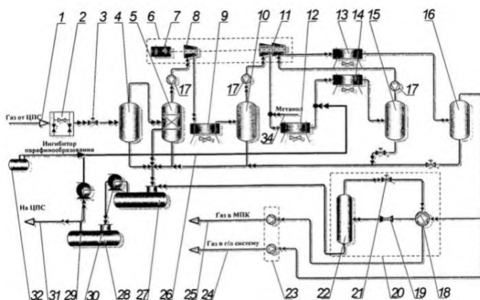
Рисунок 7.15 – Система подготовки ПНГ
