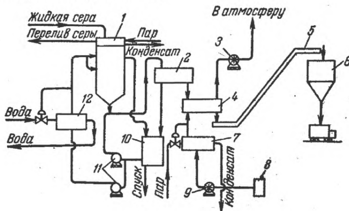
1 – гранулятор; 2 – обезвоживающий грохот; 3, 9 – вентиляторы; 4 – сушилка; 5 – подъемник гранул; 6 – бункер; 7 – воздушный подогреватель; 8 – фильтр; 10 – емкость для раствора; 11 – насосы; 12 – холодильник для раствора
