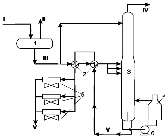
1 – входной разделитель; 2 – рекуперативный теплообменник; 3 – деэтанизатор; 4 – печь; 5 – воздушные холодильники; 6 – насос, I – нестабильный конденсат; II – газ выветривания; III – частично дегазированный конденсат; IV – газ деэтанизации; V – стабильный конденсат
