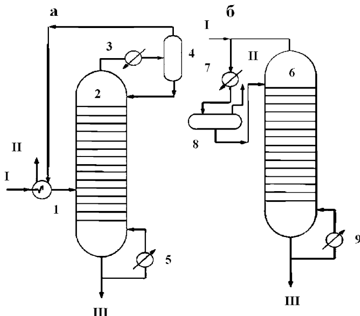
1 – теплообменник; 2 – ректификационно-отпарная колонна; 3 – конденсатор-холодильник; 4, 8 – сепараторы; 5, 9 – рубойлеры; 6 – конденсационно-отпарная колонна; 7 – холодильник с внешним холодильным циклом, I – охлажденный сырьевой газ; II – отбензиненный газ; III – ШФЛУ
