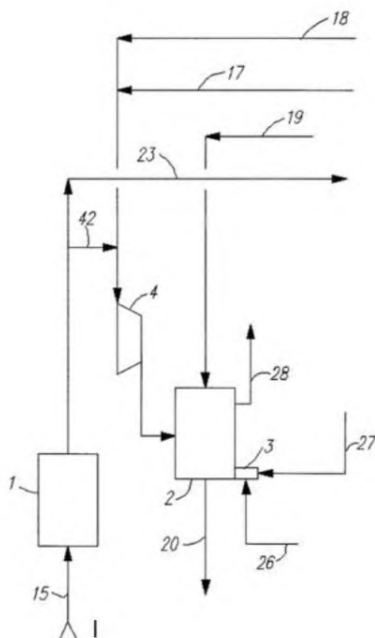
Рисунок 7.23 – Фрагмент принципиальной технологической схемы получения СЖУ из ПНГ и низконапорных малodeбитных скважин
