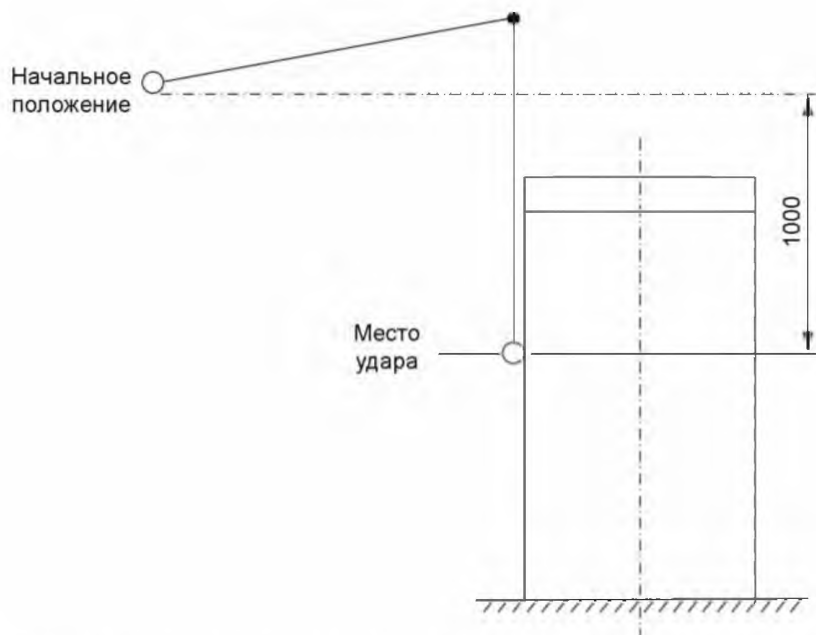
Рисунок 106b – Схема испытания устойчивости SCDB-CCO к ударному воздействию
