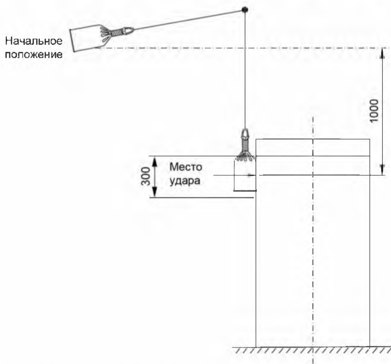
Рисунок 104б – Схема испытания устойчивости SCDB-CCO к ударной нагрузке
