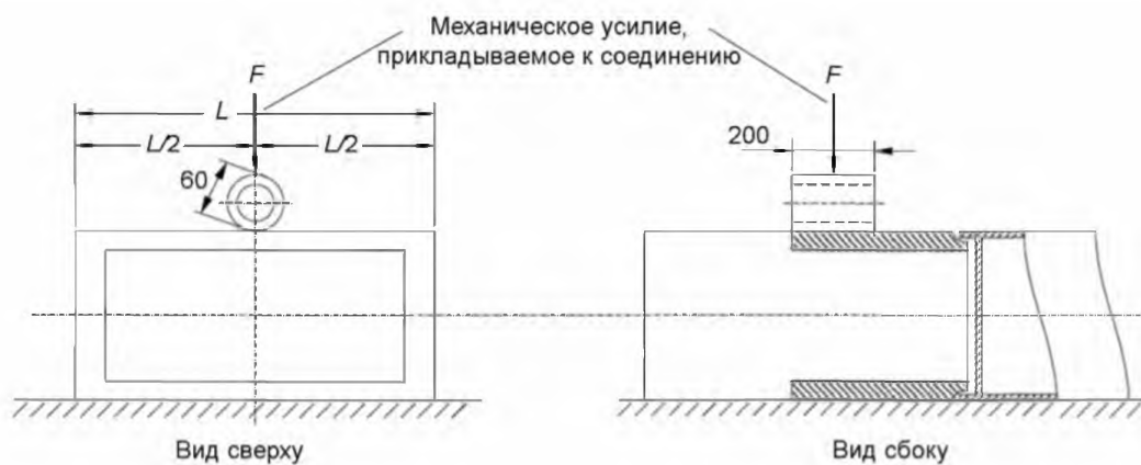
Рисунок 110 – Типовое испытательное оборудование для проверки механической прочности основания
