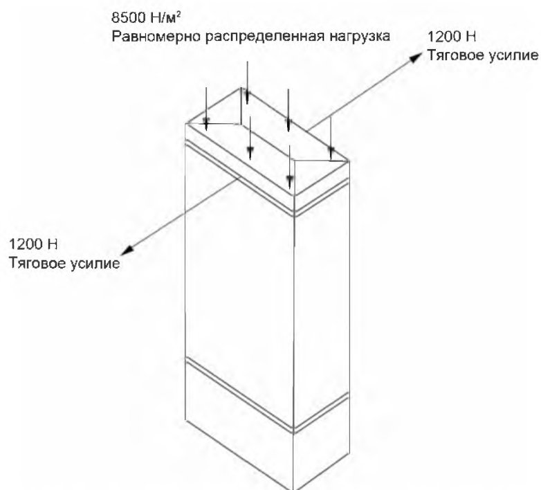
Рисунок 102 – Схема испытания устойчивости к статической нагрузке
