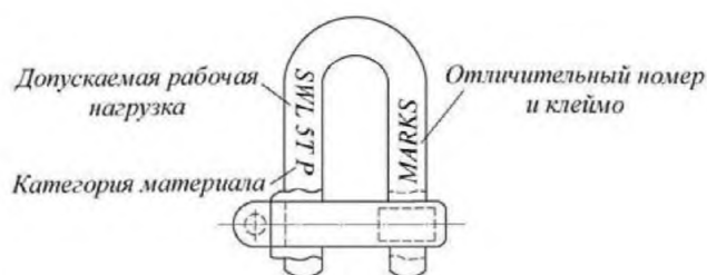
Рис. 11.2.1-3 Маркировка скобы
