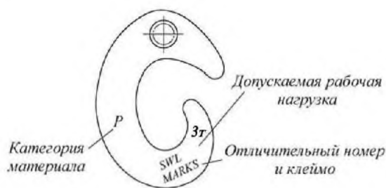
Рис. 11.2.1-1 Маркировка гака
