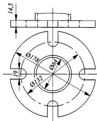
Рис. 5.1.18 Международное береговое соединение (судно)
