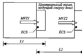
Рис. 2.2.1.2-1 Эвакуационный трап обслуживает одну главную вертикальную зону
