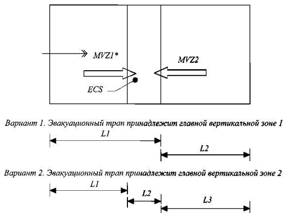
Рис. 2.2.1.2-4 Эвакуационный трап обслуживает две главные вертикальные зоны
