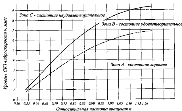
Рис. 9.9.3 Нормы вибрации винторулевых колонок
