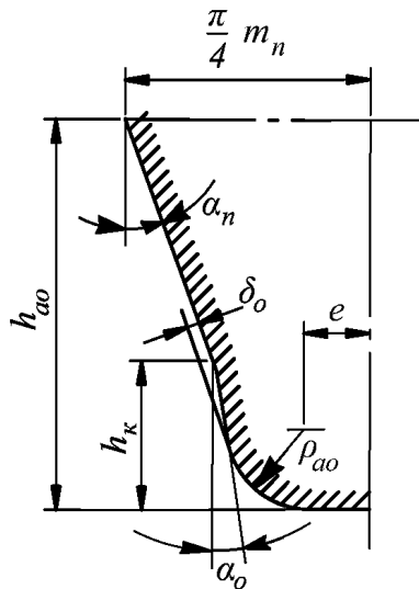
Рис. 4.2.2.7.3.2-3 Исходный производящий контур фрезы с протуберанцем
