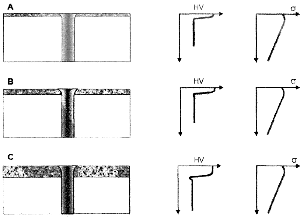
Рис. 3.2. Напряжения и твердости в индукционно закаленных краях масляных отверстий
