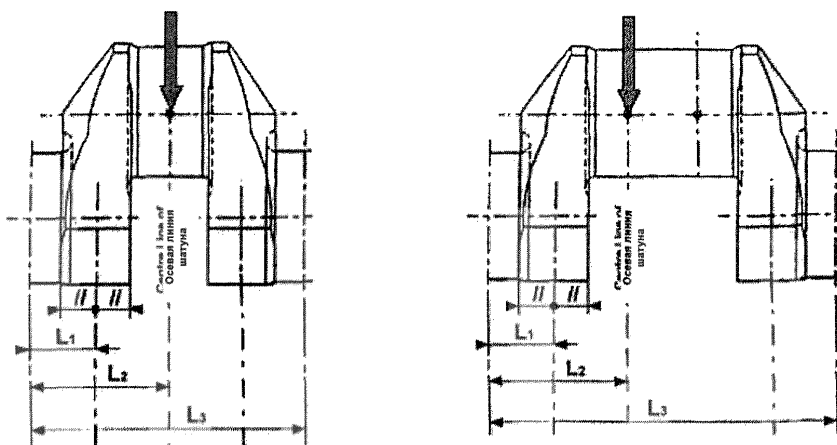
Рис. 3.4. Приложение нагрузки в случае рядного V-образного двигателя
