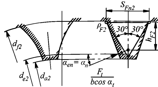
Рис. 4.2.2.7.3.2-4 К определению Y_F для случая внутреннего зацепления
