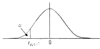
Рис. 2.5. Распределение Стьюдента
