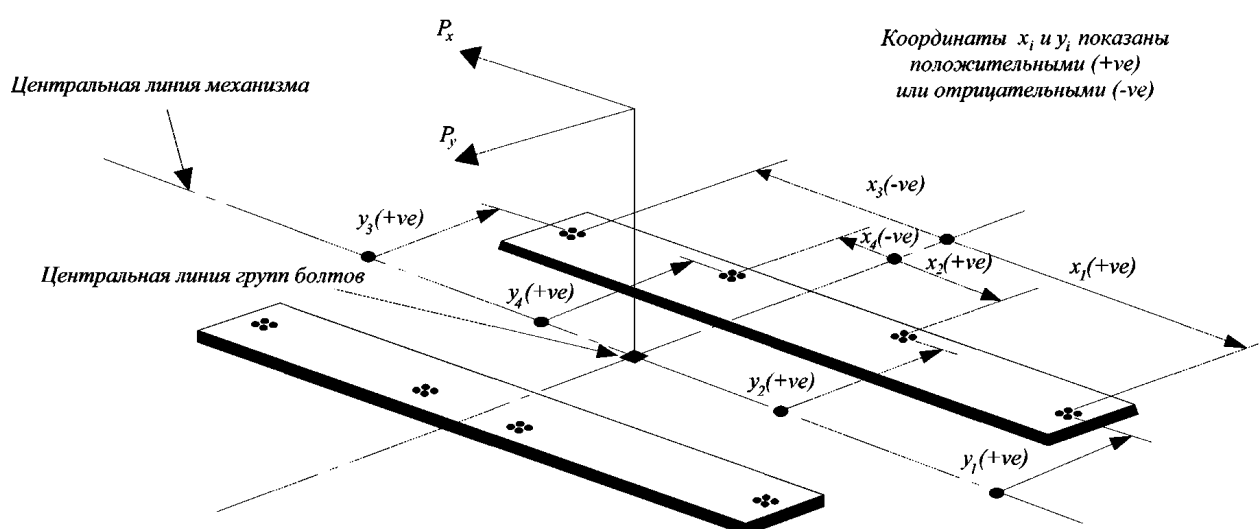
Рис. 6.3.5.4 Правило знаков
