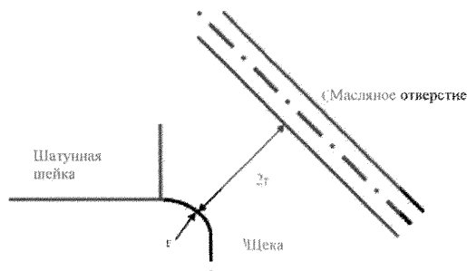
Рис. 2.1. Расстояние между масляным отверстием и галтелью
