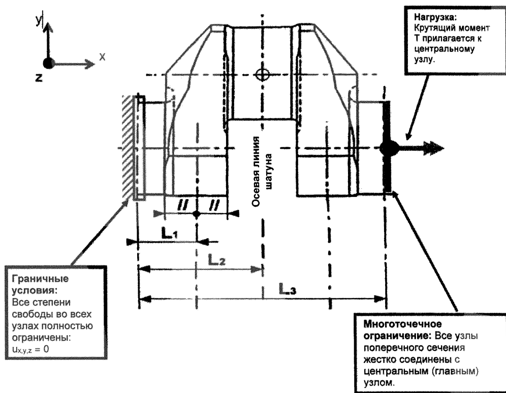
Рис. 3.1. Граничные условия и условия нагружения для случая нагружения кручением
