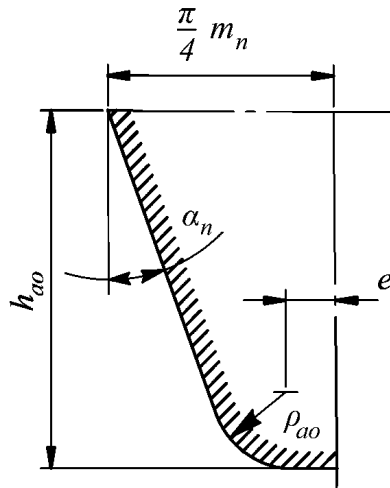
Рис. 4.2.2.7.3.2-2 Исходный производящий контур фрезы без протуберанца
