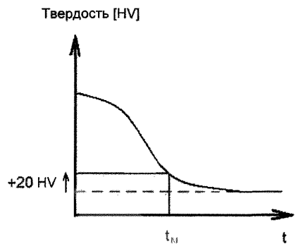
Рис. 5.1. Эскиз условной точки перехода по глубине ( t )
