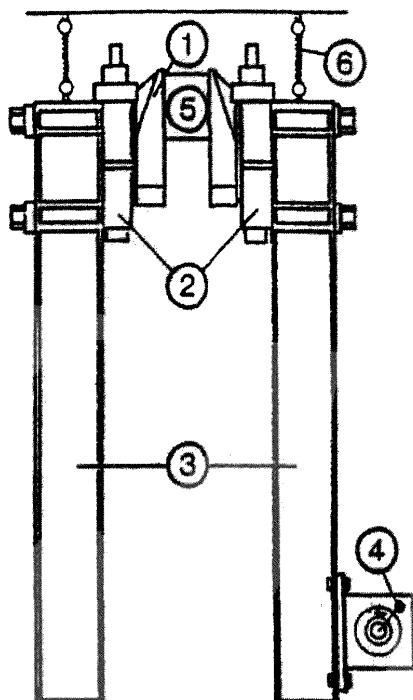
Рис. 4.2-1. Пример устройства резонансного стенда для испытания изгибной нагрузкой
