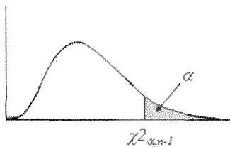
Рисунок 2.6. Распределение хи-квадрат
