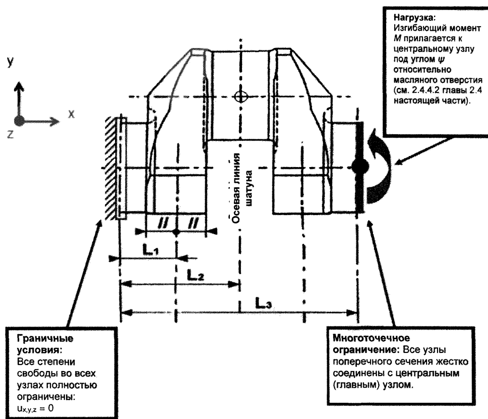
Рис. 3.2. Граничные условия и условия нагружения для случая воздействия чистым изгибом
