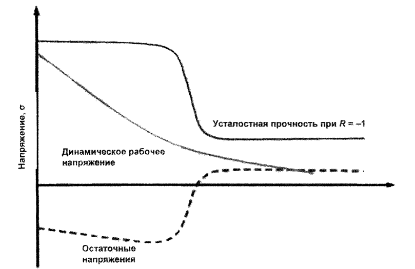
Рис. 3. Общие принципы зависимости напряжений от глубины
