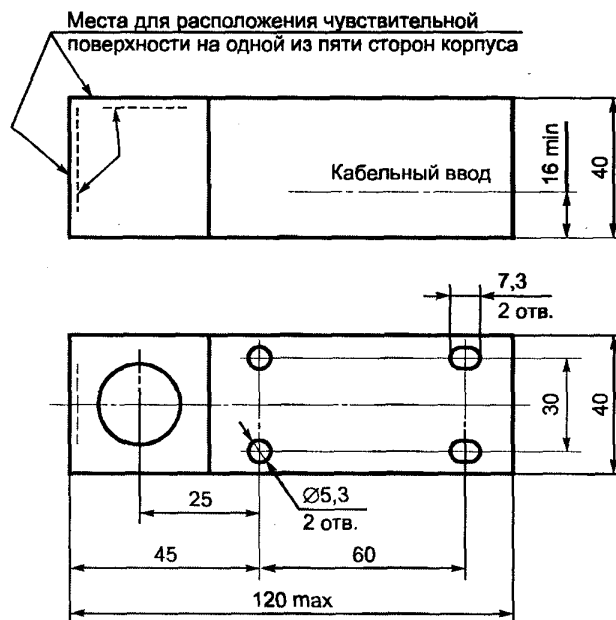
Рисунок A.1.4 (IC) – Габаритные размеры
