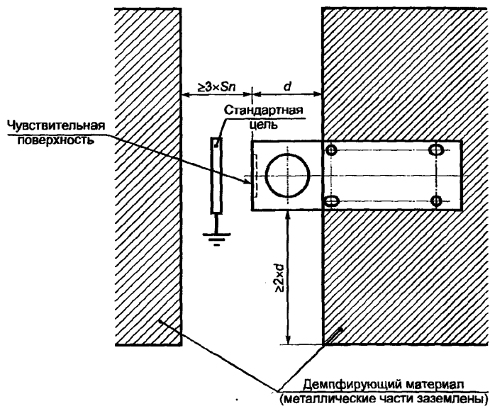
Рисунок А.2 (CC) – Установка (монтаж)
