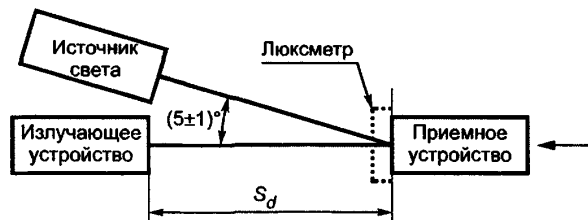
Рисунок 11а – Датчик типа Т, излучающее и приемное устройство
