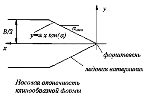
Рис. 1.2.13.2.1-1 Определение формы носовой оконечности
