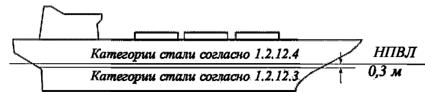
Рис. 1.2.12.3 Требования к категории стали для надводной и подводной части наружной обшивки
