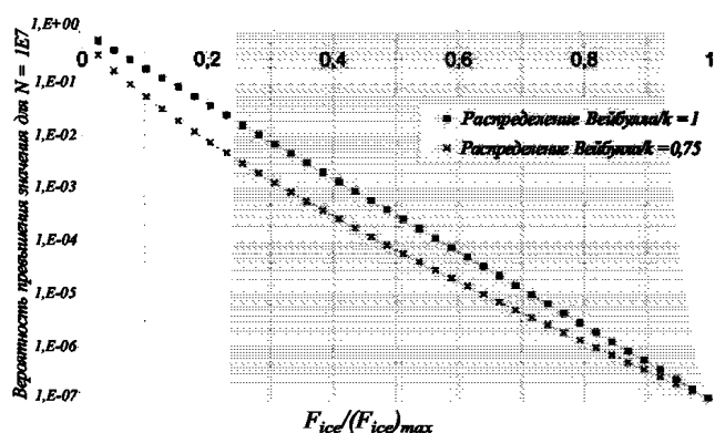
Рис.10.7.5.1.8 Распределение Вейбулла
