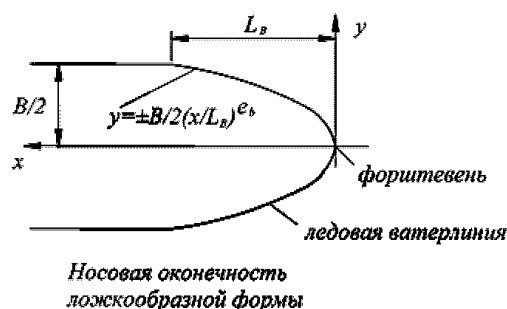
Рис. 1.2.13.2.1-1 Определение формы носовой оконечности
