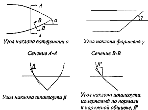
Рис. 1.2.3.2.1 Определение углов наклона
