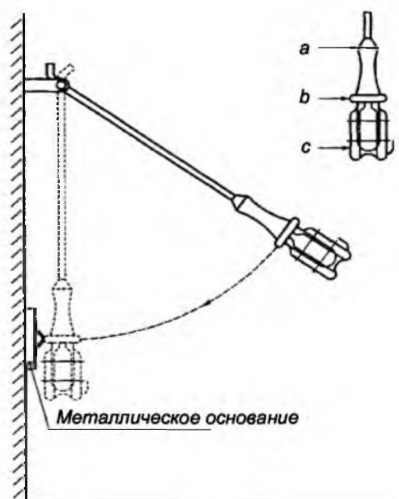
Рисунок 1 – Устройство для испытания светильников на удар
