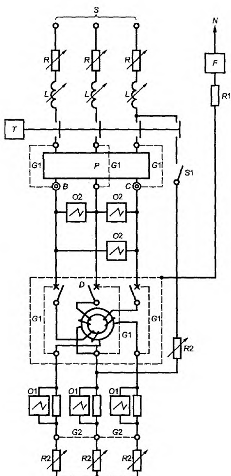
Рисунок 7 – Испытательная цепь для проверки номинальной наибольшей включающей и отключающей способности и координации с ПЗУ трехполюсного ВДТ в трехфазной сети (9.11)
