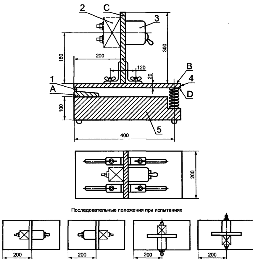
Рисунок 11 – Аппарат для испытания на механический толчок (9.12.1)
