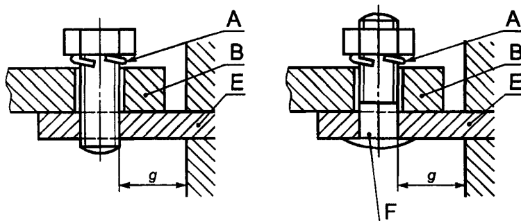
А – запорное устройство; В – кабельный наконечник или шина; Е – неподвижная часть; F – штырь
