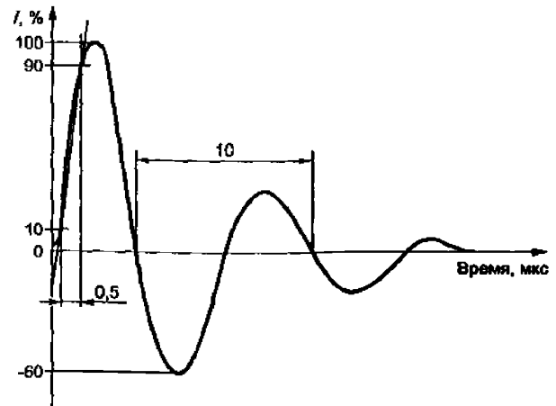
Рисунок 19а – Ток звенящей волны 0,5 мкс/100 кГц
