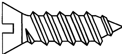
Рисунок 1 – Самонарезающий формующий винт (3.6.10)
