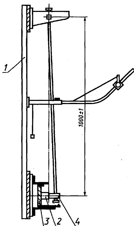
Рисунок 12 – Аппарат для испытаний на механический удар (9.12.2.1)
