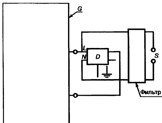
G – генератор звнящей волны; D – ВДТ; S – источник питания
