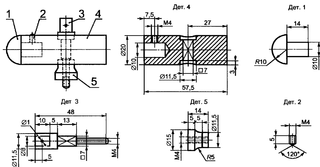
Рисунок 12 – Аппарат для испытаний на механический удар (9.12.2.1)
