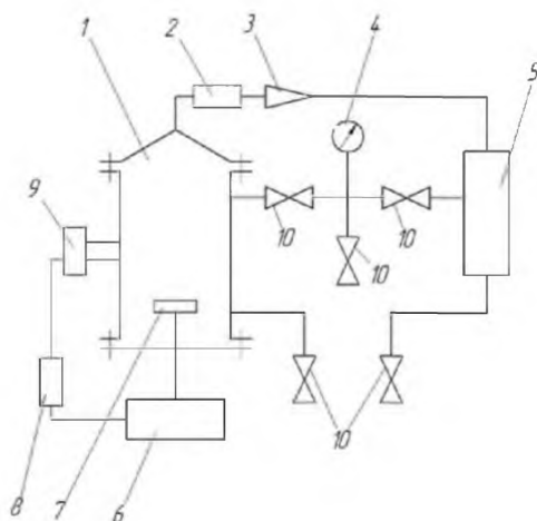
1 – реакционный сосуд; 2 – форкамера; 3 – обратный клапан; 4 – манометр; 5 – ресивер; 6 – пульт управления; 7 – источник инициирования; 8 – регистрирующая аппаратура; 9 – датчик давления; 10 – вентиль
