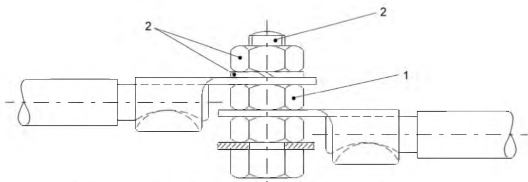
Рисунок 10 – Пример частей заземляющего зажима
