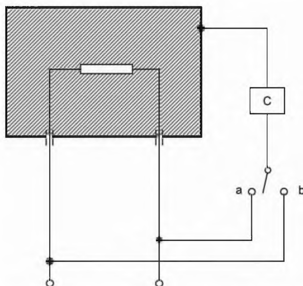
Рисунок 2 – Схема измерения тока утечки при рабочей температуре для однофазных приборов, кроме приборов класса II
