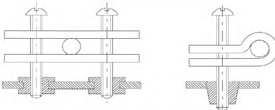
Конструкция, в которой ни одна часть не закреплена на приборе
