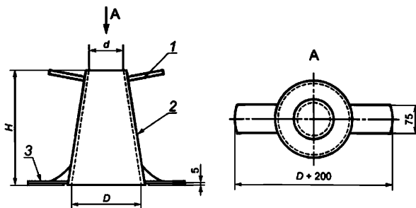
Рисунок А.1 – Конус для определения подвижности
