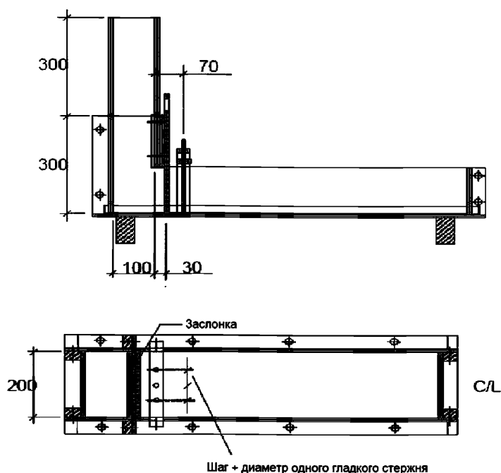
Рисунок А.7 – Конструкция L-образного ящика
