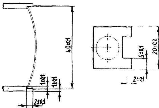
Рисунок Б. 2 - Удерживающие захваты, вид сбоку с пластинкой для испытаний в начальном положении и вид сверху, представленный без пластинки (размеры в мм)
