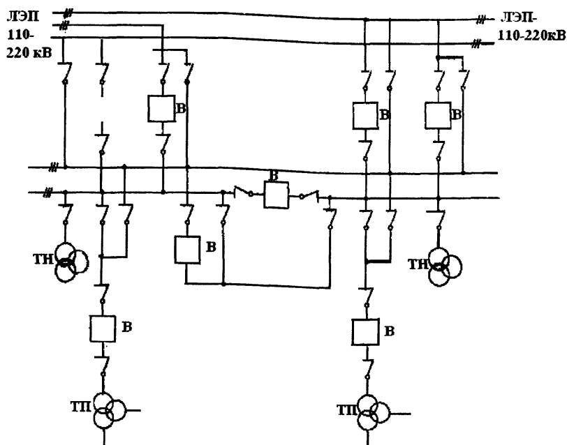
3-сурет - Жоғары кернеулі желіге тіреулік тартқыш қосалқы стансаны қосу сызбанұсқасы
