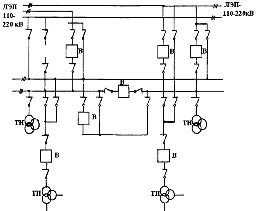
Рисунок 3 - Схема подключения опорной тяговой подстанции к сети высокого напряжения
