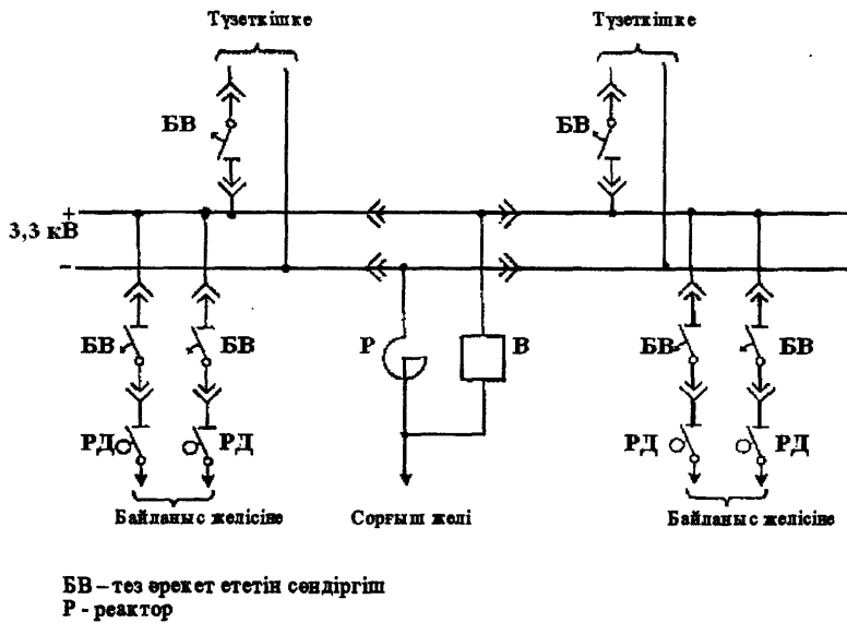
4-сурет – Айнымалы (а) және тұрақты (б) тоқтың тартқыш кернеулі тарату құрылғыларының сызбанұсқаларының үлгілері
