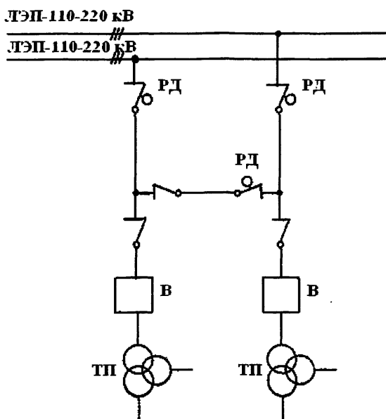
2-сурет - Жоғары кернеулі желіге дәнекерлік тартқыш қосалқы стансаны қосу сызбанұсқасы
