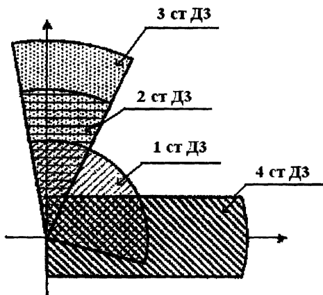
5-сурет – Айнымалы токтың байланыс желісі фидерлерін дистанциялық қорғау сатыларының әрекет ету аймақтары.
