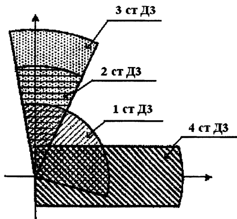
Рисунок 5 - Зоны действия ступеней дистанционных защит фидеров контактной сети переменного тока
