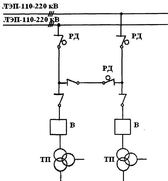
Рисунок 2 - Схема подключения отпаечной тяговой подстанции к сети высокого напряжения
