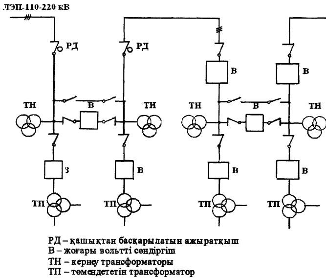
1-сурет – Жоғары кернеулі желіге транзитті тартқыш қосалқы стансаны қосу сызбанұсқасы
