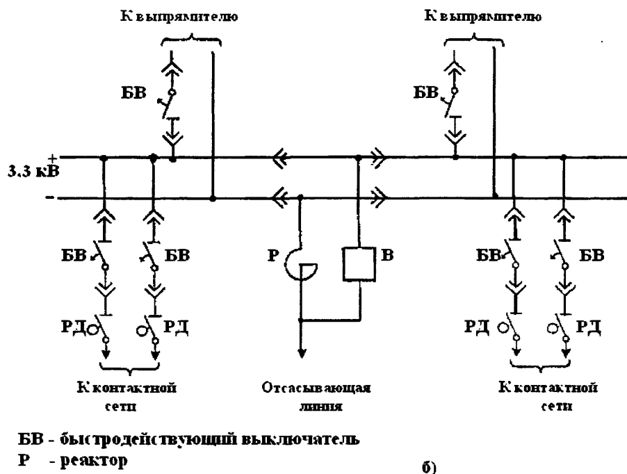
Рисунок 4 - Примеры схем распределительных устройств тягового напряжения переменного (а) и постоянного тока (б)
